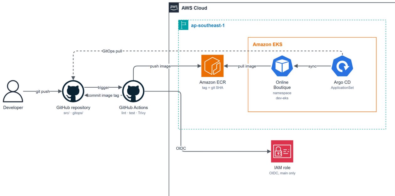
Hình 5: Từ commit tới cluster
