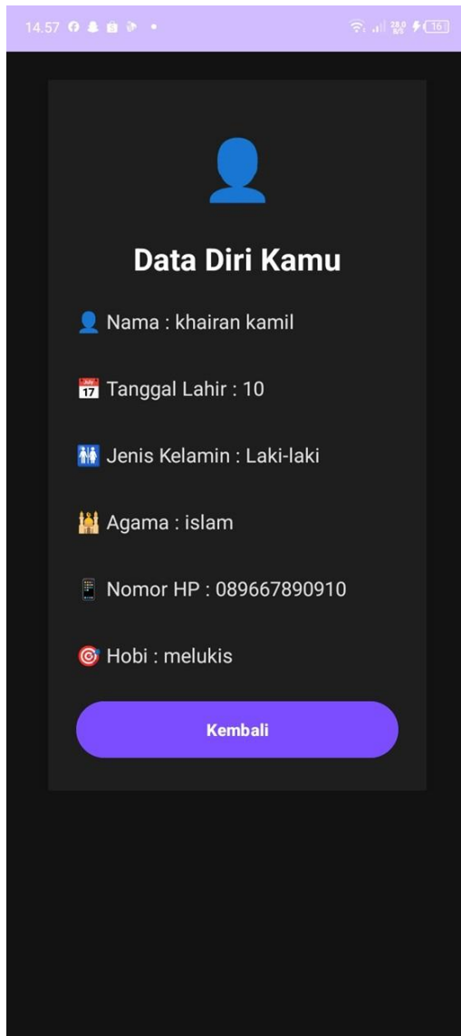
Gambar 3. Halaman Hasil
