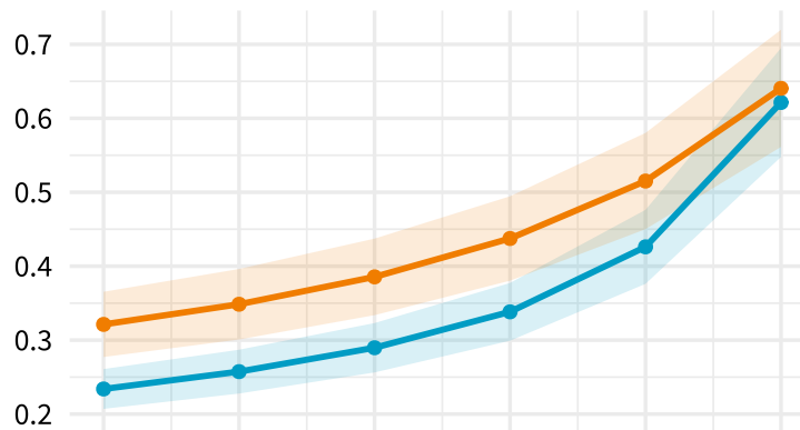
RRMSE( \Theta )
