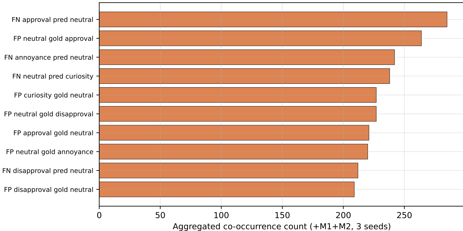
Top error motifs (test)
