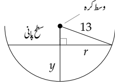
شکل ۳.۶۹: نصف کرہ ٹینگی (سوال ۳.۱۹)
