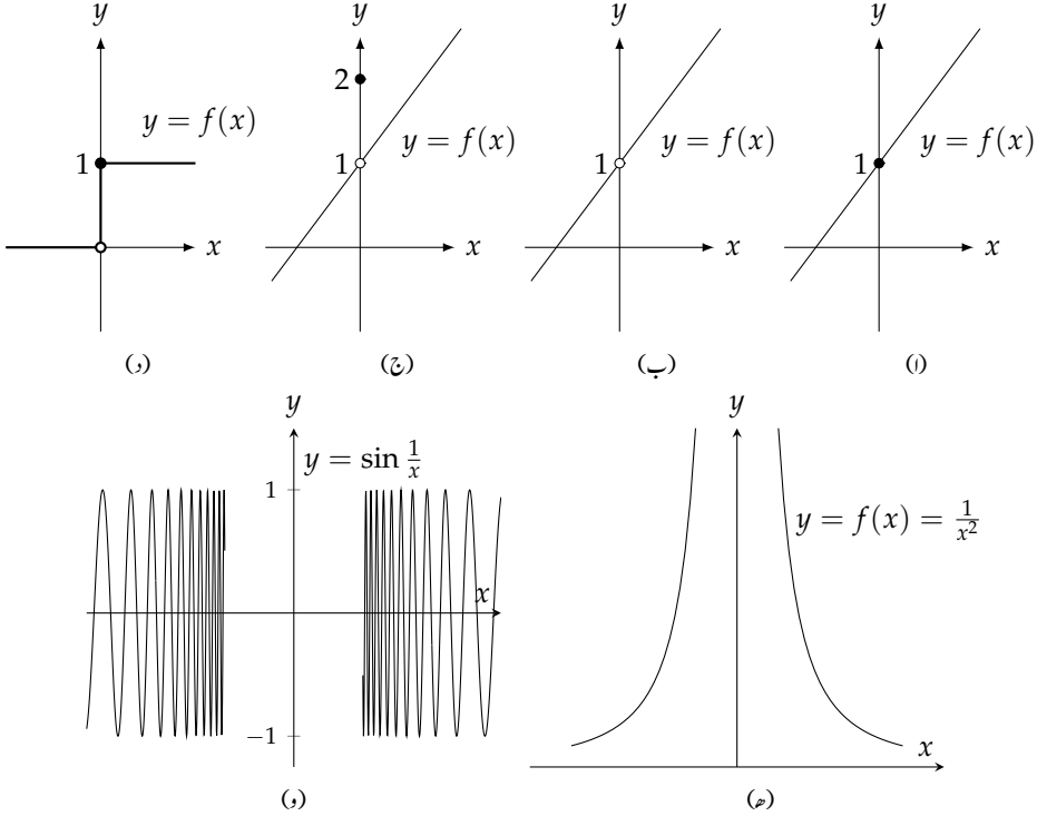
شکل ۲.۵۶: x = 0 پر تفاعل (i) استمراری ہے جبکہ (ب) تا (د) غیر استمراری ہیں۔
