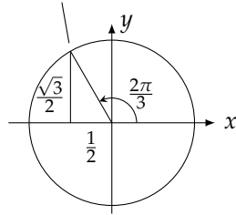
شکل ۱.۶۰: یکو نیاتی تفاعل کی قیمتیں (مثال ۱.۳)
