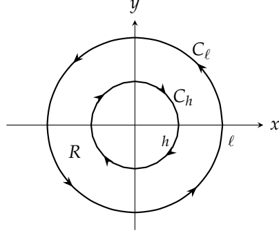
شکل ۱۵.۲۲: دکھائی گئی سرحدوں کی ہمراہ تکمل لیتے ہوئے چھلدار خط R پر مسئلہ گرین کا اطلاق کیا جاسکتا ہے (مثال ۱۵.۶)۔
