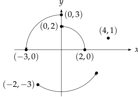
شکل ۱.۱۶: گھڑی مخالف 90^\circ گھومنا (سوال ۱.۴۸)
