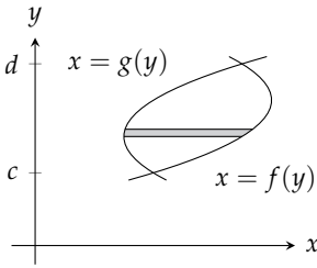
شکل ۶.۸: ان اشکال میں دایاں سرحد f اور بایاں سرحد g ہو گا لہذا f(y) - g(y) غیر منفی ہو گا۔
