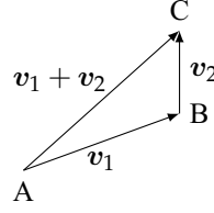
شکل ۱۱.۳: سمتیات v_1 اور v_2 کا مجموعہ۔
