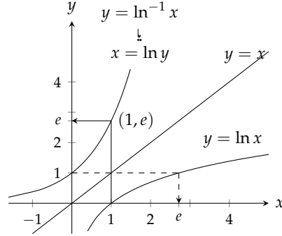
شکل ۷.۲۶: تفاعل y \ln x اور تفاعل y = \ln^{-1} x ۔ عدد e سے مراد 1 \ln^{-1} ہے۔
