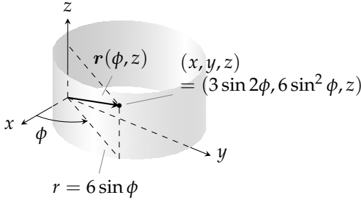
شکل ۱۵.۶۲: تکلی محدود استعمال میں مثال ۱۵.۳ کے بیلیں کا مقدار معلوم روپ۔
