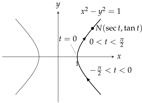
شکل ۱۰.۳۰: قطع زائدرہ (مثال ۱۰.۷)
