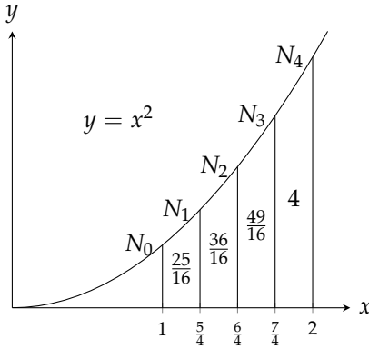
شکل ۵.۲۳: ذوزنقہ قاعدہ متعلق y = x^2 کا رقبہ کچھ زیادہ دیتا ہے۔
