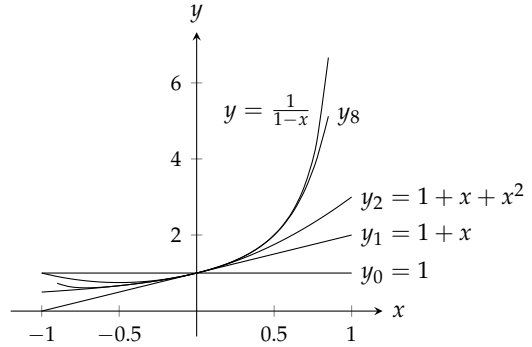
شکل ۹.۲۳: f(x) = \frac{1}{1-x} اور اس کی چار تخمینی رکنیاں (مثال ۹.۱)۔
