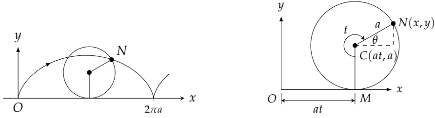
شکل ۱۰.۴۱: پیسے کے محیط پر نقطے کا مقام اور تندیر۔
