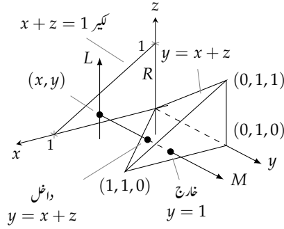
شکل ۱۴.۳: چو سطح (مثال ۱۴.۲)
