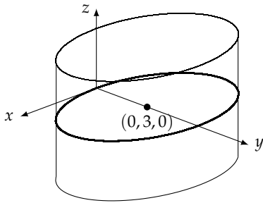
شکل ۱۱.۶۵: نکلی نمائے مثال ۱۱.۵
