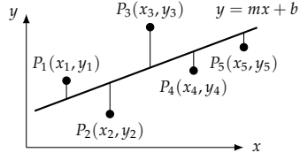
شکل ۱۳.۱۴: غیر ہم خطی نقاط پر سیدھا خط بٹھانے کے لئے ہم وہ لکیر منتخب کرتے ہیں جس میں انتظامی فرق کے مربع کا مجموعہ کم سے کم ہو۔
