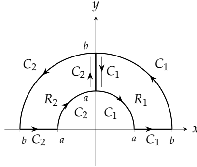
شکل ۱۵.۲۰: خطہ R_1 اور R_2 کو ملا کر خطہ R حاصل کیا گیا ہے۔
