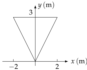
شکل ۶.۱۳۳: مثلث الساقین (سوال ۹)
