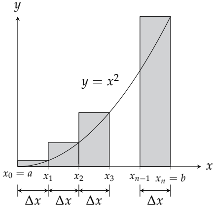
شکل ۵.۳۲: ریمان مجموعوں کے مستطیل (مثال ۹)
