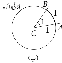
شکل ۱.۴۸: ریڈین کی تعریف
