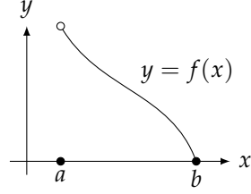
(ا) ایک آخری نقطہ پر غیر استمراری
