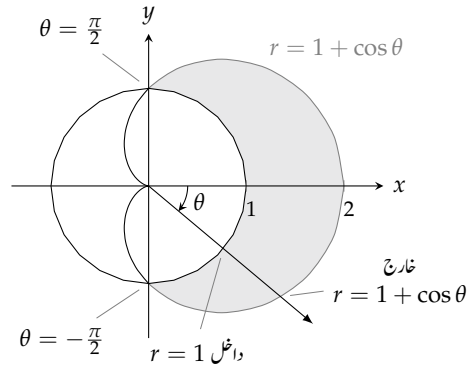
شکل ۱۴.۳: دائرہ اور قلب نما (مثال ۱۴.۱)
