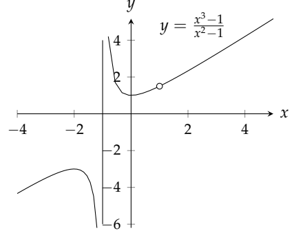
شکل ۴.۶۸: منحنی f(x) = \frac{x^3-1}{x^2-1} کی x = 1 پر عدم استمرار قابل ہٹاؤ ہے لہذا اس کی صرف x = -1 پر متقاربی خط ہو گا۔
