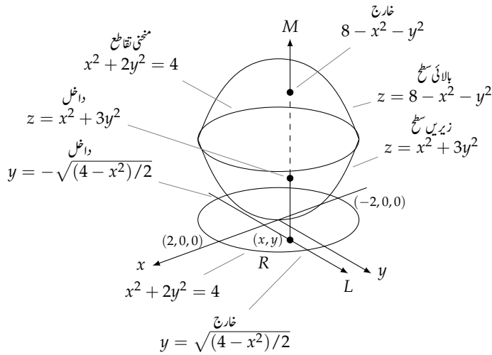
شکل ۱۴.۳۲: دو سطحوں کے بیچ حجم (مثال ۱۴.۱)
