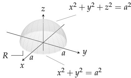
شکل ۱۵.۵۵: مستقل کمیتی کثافت کی باریک چادر کا نصف کروی خول (مثال ۱۵.۵)۔
