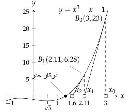
شکل ۴.۱۰۰: جنر حاصل کرنے کی خاطر x = \frac{1}{\sqrt{3}} کے دائیں جانب کسی بھی نقطہ x_0 سے شروع کیا جا سکتا ہے۔
