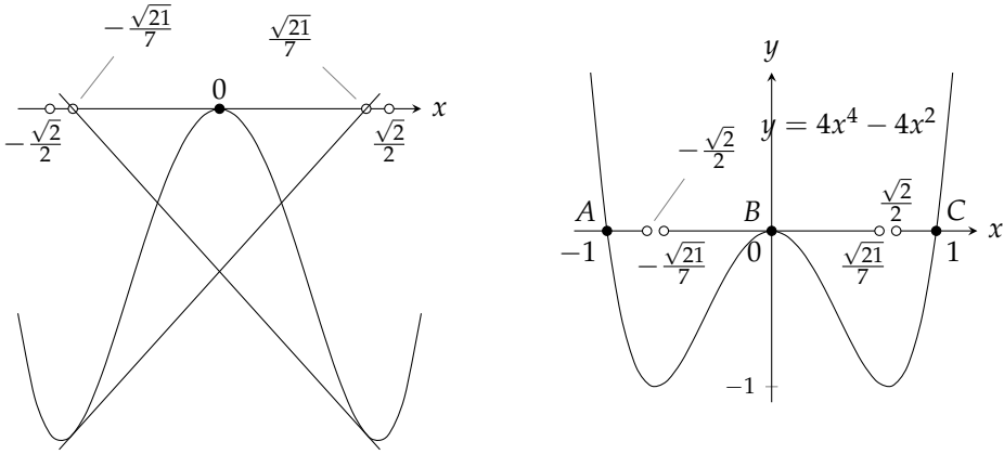
شکل ۴.۱۰۵: ترکیب نیوٹن ابتدی کا شکار ہے۔
