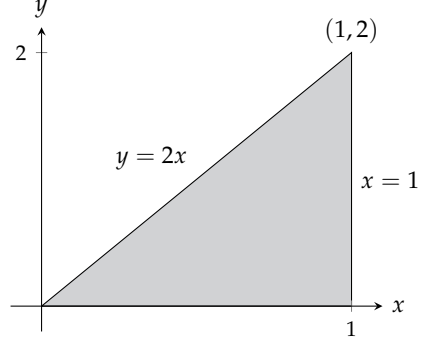
شکل ۱۴.۳: خطہ برائے مثال ۱۴.۴
