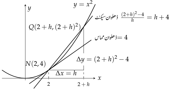
شکل ۲.۴۳: قطع مکانی کا مماس (مثال ۲.۱)
