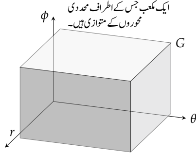
(c) کارتیسی r\theta\phi فضا۔
