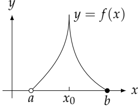
(ج) [a, b] پر استمراری لیکن کسی اندرونی نقطہ پر نا قابل تفریق
