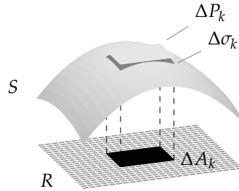
شکل ۱۵.۴۶: مماسی چادر Delta P_k تخمیناً رقبہ Delta A_k سے اوپر سطحی رقبہ Delta sigma_k کو ظاہر کرتی ہے۔
