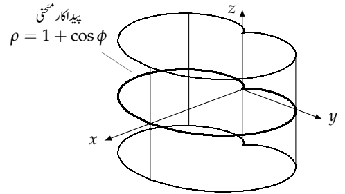
شکل ۱۱.۶۴: قلب نما مساوات \rho = 1 + \cos \phi فضا میں نیکی کو ظاہر کرتی ہے جس کا عمودی تراش محور z کو قائمہ ہے (مثال ۱۱.۲)۔
