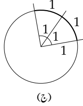
شکل ۱.۴۸: ریڈین کی تعریف
