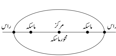
شکل ۱۰.۵: ترخیم پر اہم نقطے۔
