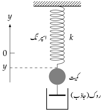
شکل ۸.۴: اسپرنگ، کمیت اور جاذب کا قسری نظام (سوال ۴۱ اور سوال ۴۲)۔
