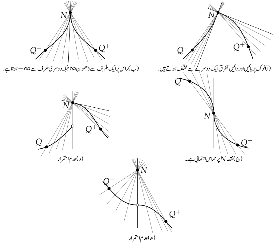
شکل ۸.۳: ان نقطوں کی پہچان جہاں تفاعل ناقابل تفریق ہو گا۔
