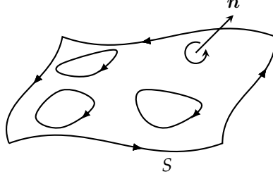
شکل ۱۵.۷: سوراخ دار سمت بند سطوح پر بھی مسئلہ سٹوکس کا اطلاق ہوتا ہے۔
