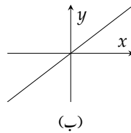
شکل ۱۲.۳: تفاعل کے تفرق
