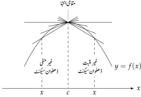
شکل ۷. ۳: اندرونی نقطہ پر مقامی انتہا پر ڈھلوان صفر ہوگا (مسئلہ ۲)۔
