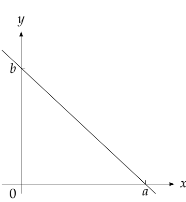
شکل ۱.۱۲: غیر انتصابی اور غیر افقی خط کے محوری قطعات
