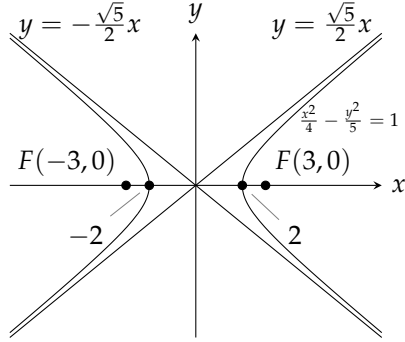
شکل ۱۰.۱۴: قطع زائد (مثال ۴)
