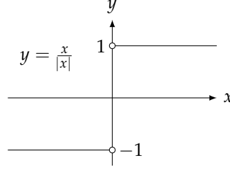
شکل ۲.۳۹: مبدا پر بائیں ہاتھ حد اور دائیں ہاتھ حد مختلف ہیں۔
