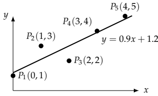
شکل ۱۳.۱۵: کٹر مربع خط۔
