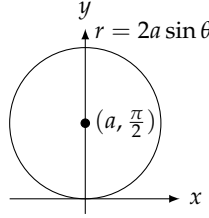
شکل ۱۰.۳: کارتیسی محور پر مرکوز والے دائروں کے قطبی مساوات۔
