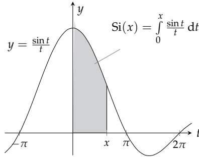
شکل ۵.۷: تفاعل سائن تکمیل (سوال ۳۲)
