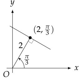
شکل ۱۰.۲: خط برائے مثال ۱
