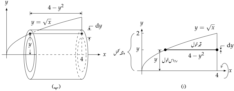
شکل ۶.۱۰: محور x کے گرد طواف (مثال ۲)
