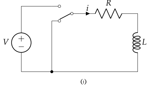
شکل ۷.۲۶: سلسلہ وار مزاحمت، امالہ برقی دور (مثال ۹)
