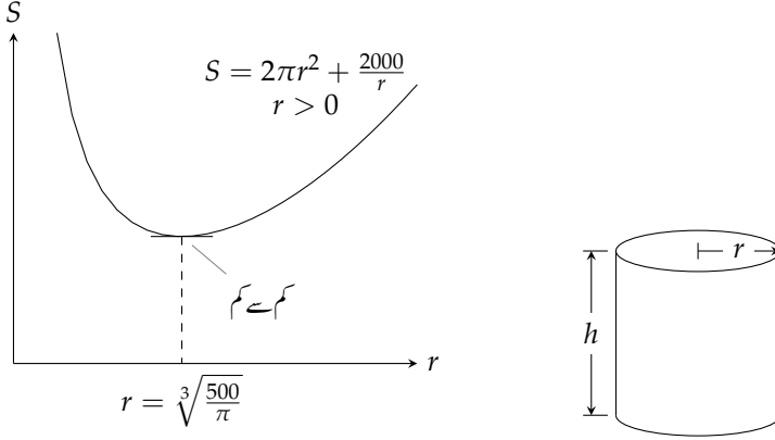
شکل ۳.۴: ٹین کا ڈبہ (مثال ۲)
