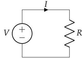
شکل ۲.۳۳: قانون اوہم (سوال ۵۶)
