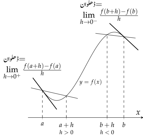
شکل ۷.۳: وقفہ کے آخری سر نقطوں پر تفرق یک طرفہ ہوں گے۔
