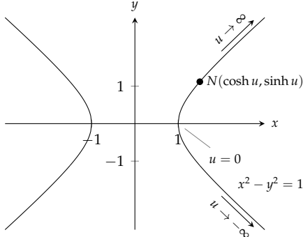
شکل ۷.۲۳: قطع زائد تفاعل کے نام کی وجہ (سوال ۸۶)
