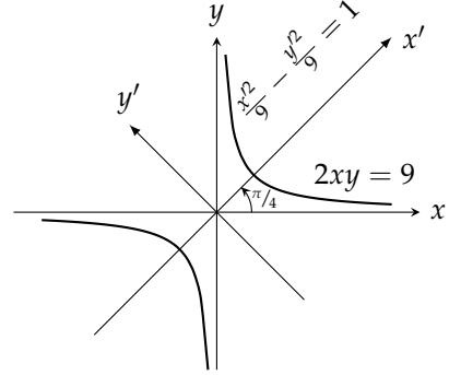
شکل ۱۰.۳۱: نئے محور x' اور y' میں قطع زائد کی مساوات (مثال ۱)
