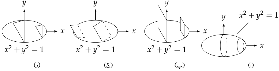
شکل ۶.۳۱: عمودی تراش برائے سوال ۱
