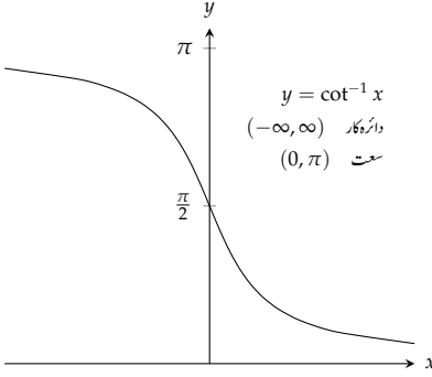
شکل ۷.۲۰: y = \cot^{-1} x ترسیم
