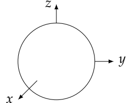
(ل) مستقل رداس کرہ دیتا ہے۔
