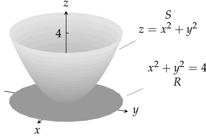
شکل ۱۵.۴۸: اس قطع مکانی سطح کارقبہ مثال میں حاصل کیا گیا ہے۔
