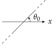
شکل ۱۰.۶۰: قطبی محدود پر \theta = \theta_0 سیدھی لکیر ہے۔
