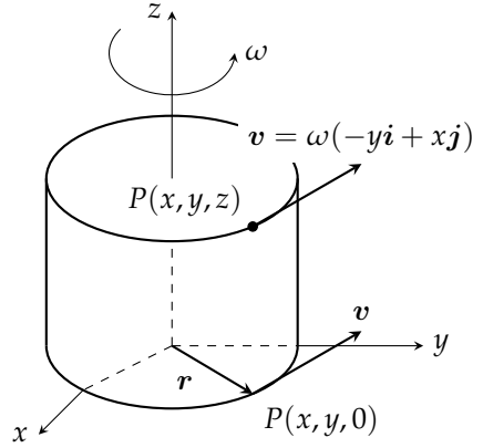
شکل ۱۵.۷.۶: مستوی xy میں مثبت (غلاف گھڑی) مستقل زاویائی سمتی رفتار \omega کے ساتھ، مستوی xy کے متوازی سیال برقرار گھوم رہا ہے (مثال ۴)۔
