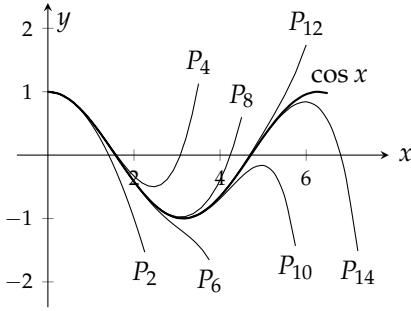
شکل ۹.۲: کوسائن اور اس کی ٹیلر کثیر رکنیاں (مثال ۳)
