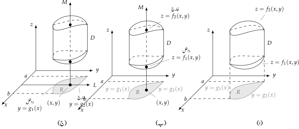
شکل ۱۴.۳۱: تہر انکملاٹ کی حدوں کی تلاش۔
