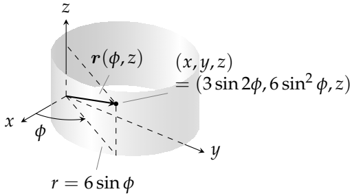
شکل ۱۵.۶۲: تکلی محدود استعمال میں مثال ۳ کے پیلن کا مقدار معلوم روپ۔
