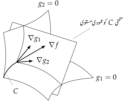
شکل ۱۳.۵: چونکہ \nabla g_1 = 0 سطح g_1 = 0 کو عمودی ہے اور \nabla g_2 = 0 سطح g_2 = 0 کو عمودی ہے لہذا سمتیت \nabla g_1 اور \nabla g_2 منحنی C کے عمودی مستوی میں پائے جاتے ہیں۔
