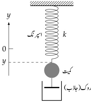
شکل ۸.۴: اسپرنگ، کمیت اور روک (جاذب) کا قسری نظام (سوال ۴۱ اور سوال ۴۲)۔
