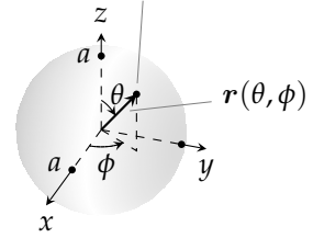
شکل ۱۵.۶۱: کروی محدود استعمال میں مثال ۲ کے کرہ کا مقدار معلوم روپ۔
