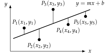
شکل ۱۳.۱۶: غیر ہم خطی نقاط پر سیدھا خط بٹھانے کے لئے ہم وہ کلیئر منتخب کرتے ہیں جس میں انتصابی فرق کے مرلج کا مجموعہ کم سے کم ہو۔
