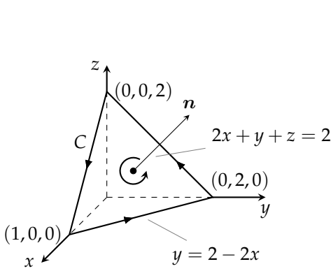
شکل ۱۵.۷.۵: سطح برائے مثال ۵
