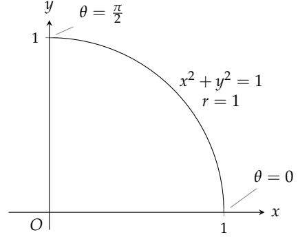
شکل ۱۴.۲۸: قطبی محدود میں یہ خطہ 0 \leq \theta \leq \frac{\pi}{2} , 0 \leq r \leq 1 ہے۔
