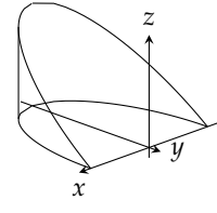
شکل ۱۴.۴۱: خاکہ برائے سوال ۲۶
