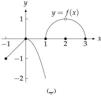
شکل ۲.۹: ۲۰ اشکال برائے سوال ۱۳ اور سوال ۴
