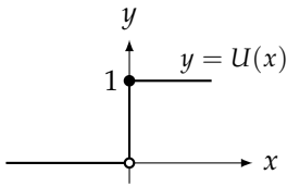
شکل ۲.۵۹: یہ تفاعل مبداء پر دائیں استتاری ہے
