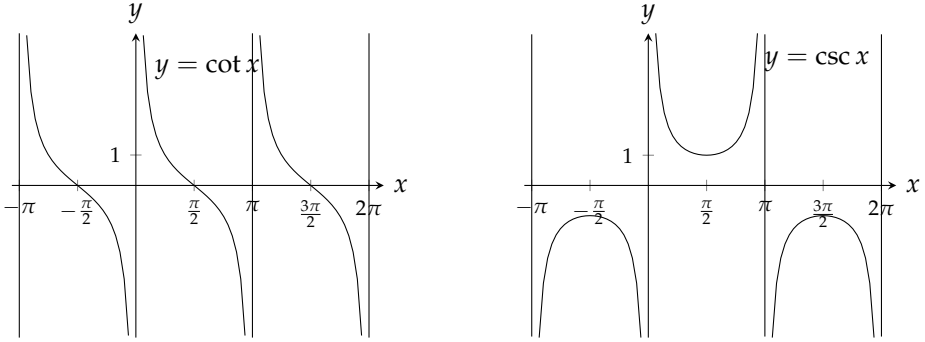
شکل ۴.۶۵: انتظامی مقارب (مثال ۷)
