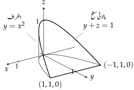
شکل ۷.۱۴: خاکہ برائے سوال ۲۱
