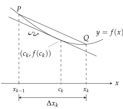
شکل ۶.۴۶: نقطہ (c_k, f(c_k)) پر ماس اور قطع متوازی ہیں۔
