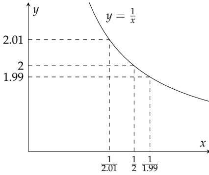
شکل ۲.۳۰: ترتیبم برائے سوال ۱۴
