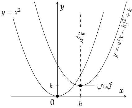
شکل ۱.۳۰: قطع مکانی y = ax^2 , a > 0 کو h کا نیا دائیں اور k کا نیا اوپر منتقل کیا گیا ہے
