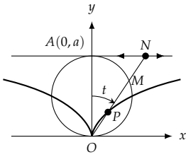
شکل ۱۰.۵: تریسہات برائے سوال ۳۵
