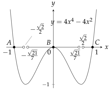
شکل ۴.۱۰۵: ترکیب نیوٹن اتری کا شکار ہے۔
