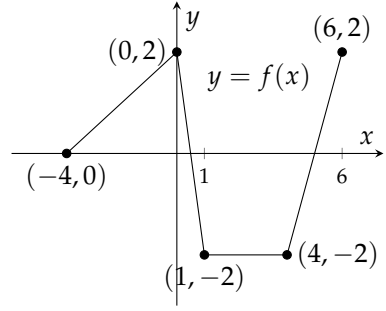
شکل ۱۴: ۳.۱۴: ترسیم برائے سوال ۳۱
