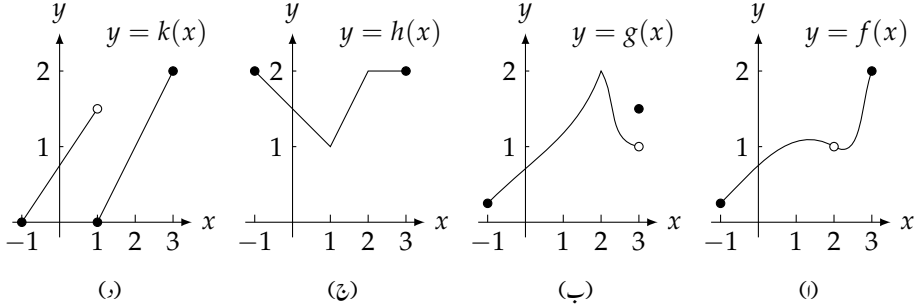
شکل ۲.۶۸: ۳ سوال ۱ تا سوال ۴
