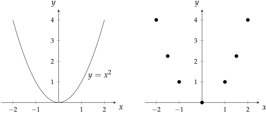
شکل ۱.۲۰: y = x^2 تفاعل کی ترسیم (مثال ۲)
