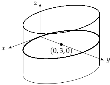
شکل ۱۱.۶۵: نیکی نمائے مثال ۵
