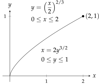
شکل ۶.۴۹: معنی برائے مثال ۲
