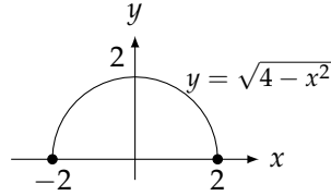
شکل ۲.۵۸: پورے دائرہ کار کے پر نقطہ پر استتاری
