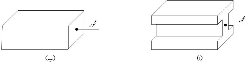
شکل ۱۴.۱۹: دونوں شبیر کا رقبہ عمودی تراش ایک جیسا ہے لیکن شبیر-اکا جمودی معیار اثر زیادہ ہے لہذا شبیر-از زیادہ اکڑ ہو گا۔
