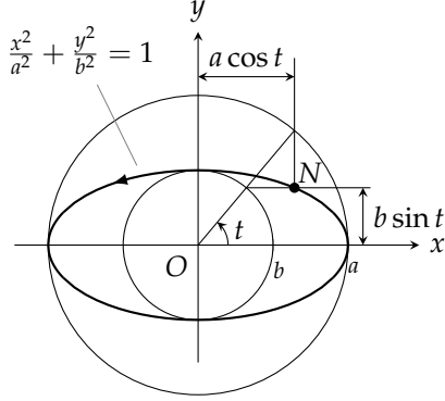
شکل ۱۰.۳۹: ترخیسی راہ (مثال ۵)
