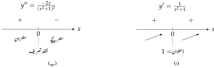
شکل ۵.۳: منحنی کی اتار چڑھاؤ اور مقعر (مثال ۴)
