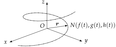
شکل ۱۲.۱: فضائیں متحرک ذرہ کا تعین کر سکتی ہیں۔ \vec{r} = \vec{ON} متغیر t کا تفاعل ہوگا۔
