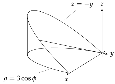
شکل ۱۴.۸۱: جسم برائے شکل ۱۴.۶
