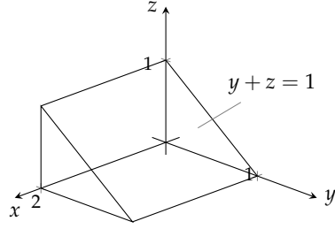
شکل ۱۴.۳۶: منشور کے حجم کی چھ بارہا تہرا کھمبات مثال ۳ میں دیے گئے ہیں۔
