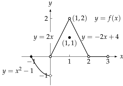
شکل ۲.۶۹: ۱۰ سوال ۵ تا سوال ۱۰
