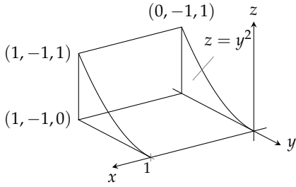
شکل ۷.۱۴: خاکہ برائے سوال ۲۲
