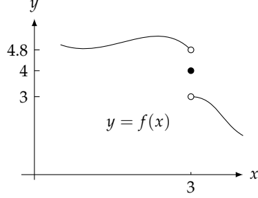
شکل ۲.۳۷: ترسیم برائے سوال ۵۹
