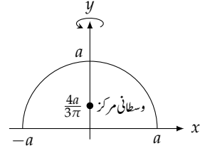
شکل ۲.۱۴۳: نصف کرہ کا وسطانی مرکز (مثال ۳)
