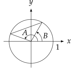
شکل ۱.۷: اشکال برائے سوال ۵۳
