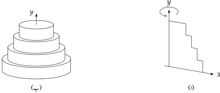
شکل ۶.۵۶: تکلی جسم طواف
