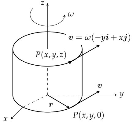
شکل ۱۵.۷.۶: مستوی xy میں مثبت (علاف گھڑی) مستقل زاویائی سمتی رفتار omega کے ساتھ، مستوی xy کے متوازی سیال برقرار گھوم رہا ہے (مثال ۴)۔
