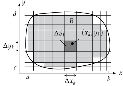
شکل ۱۴.۱۵: ایک خطے کے رقبے کی تلاش میں پہلا قدم خطے کی اندرون کی خانہ بندی ہے۔
