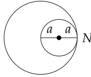
شکل ۱۰.۵: تہدویر برائے سوال ۳۴
