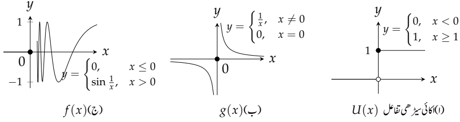
شکل ۷.۲: اشکال برائے مثال ۹
