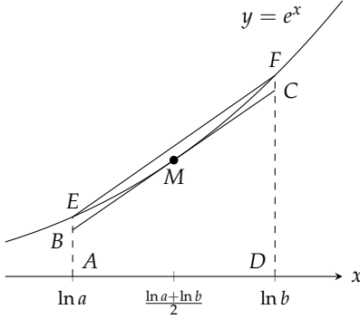
شکل ۴.۳۰: ترتیب برائے سوال ۸۲
