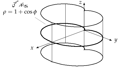
شکل ۱۱.۶۴: قلب نما مساوات \rho = 1 + \cos \phi فضا میں نیکی کو ظاہر کرتی ہے جس کا عمودی تراش محور z کو قائمہ ہے (مثال ۲)۔
