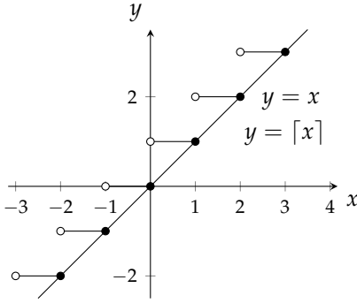
شکل ۱.۲۷: عدد صحیح چھت تقاضا (مثال ۹)
