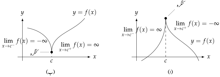
شکل ۴.۴: سنگمرہ، مقامی زیادہ سے زیادہ یا مقامی کم سے کم نقطہ ہو سکتا ہے۔
