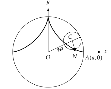
شکل ۱۰.۵: ستارہ نما۔ سوال ۳۳
