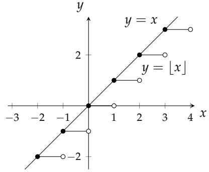
شکل ۱.۲۶: عدد صحیح زمین تقاضا (مثال ۸)
