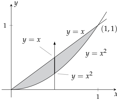
شکل ۱۴.۱۶: قطع مکانی اور لکیر کے بیچ رقبہ (مثال ۱)۔
