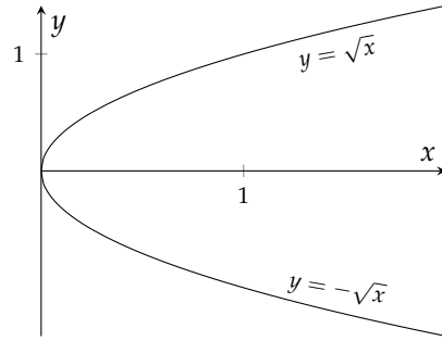
شکل ۱.۳۹: تقابل y = \sqrt{x} اور y = -\sqrt{x} کی ترسیم مبدا پر ملتے ہیں اور مساوات x = y^2 کی ترسیم دیتے ہیں (مثال ۱۱)
