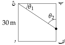
شکل ۳.۷.۷: بچوں کا کھیل (سوال ۳۷)
