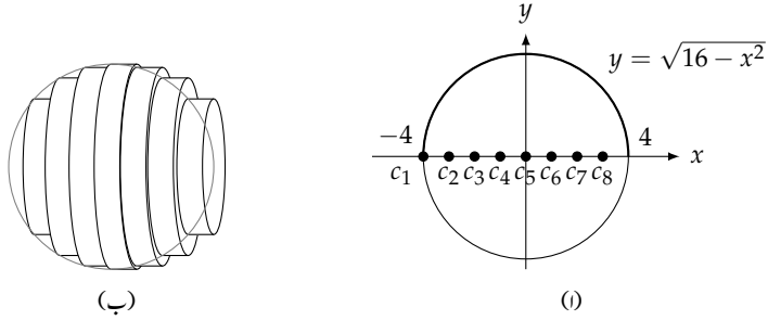
شکل ۵.۱۵: نصف دائرہ y = \sqrt{16 - x^2} کو x محور کے گرد گما کر کرہ حاصل کیا جاتا ہے (مثال ۴)۔
