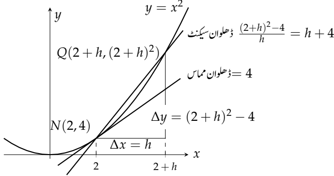
شکل ۲.۷۳: قطع مکانی کا مماس (مثال ۱)
