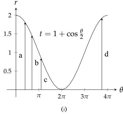
شکل ۱۰.۶۶: ترسیمات برائے مثال ۳
