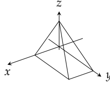
شکل ۱۴.۳۹: خاکہ برائے سوال ۲۴
