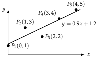
شکل ۱۳.۱۵: کٹر مرلج خط۔
