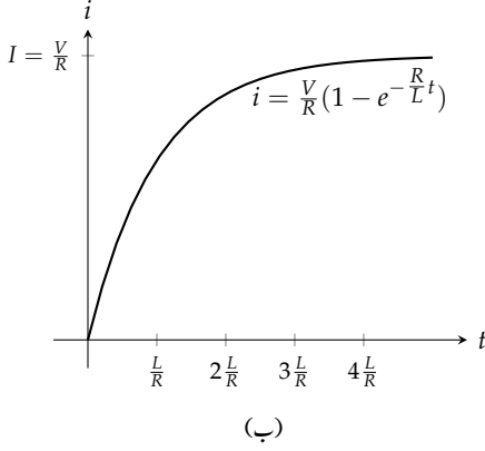
شکل ۶۸. ۷: سلسلہ دار مزاحمت و امالہ برقی دور (مثال ۸۹. ۷)
