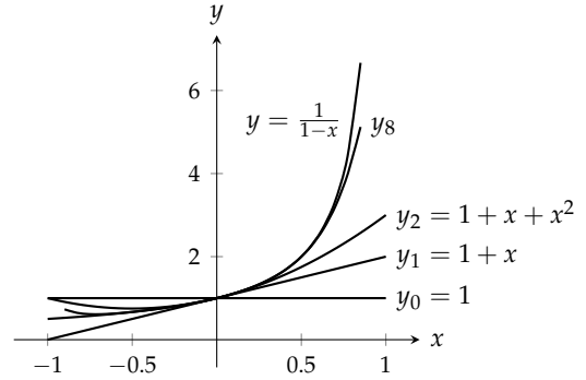
شکل ۹.۲۴: تقابل f(x) = \frac{1}{1-x} اور اس کی چار تخمینی کثیر رکنیاں (مثال ۹.۴۷)۔
