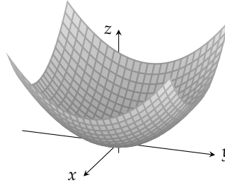
شکل ۱۳.۶۰: تعامل f(x, y) = x^2 + y^2 کی ترسیم قطع کافی سطح z = x^2 + y^2 ہے۔ اس تعامل کا ایک فاصل نقطہ پایا جاتا ہے، جو مبداء پر ہے اور جس پر مقامی اقل قیمت 0 پائی جاتی ہے۔
