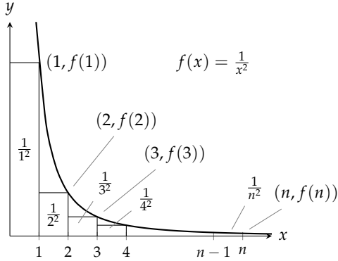
شکل ۹.۲۱: رقبہ کا موازنہ (مثال ۹.۲۹)
