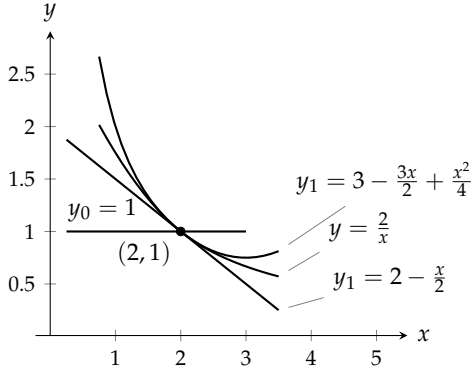
شکل ۹.۲۵: تقابل f(x) = \frac{2}{x} اور اس کی ابتدائی تین تخمینی رکنیاں (مثال ۹.۴۸)۔
