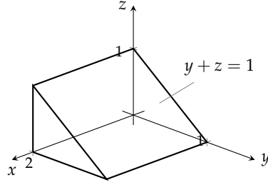
شکل ۱۴.۳۴: منشور کے حجم کی چھ بارہا تکملات مثال ۱۴.۱۶ میں دیے گئے ہیں۔
