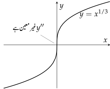
شکل ۴.۳: نقطہ تصریف پر y'' غیر معین ہے (مثال ۴.۱۶)
