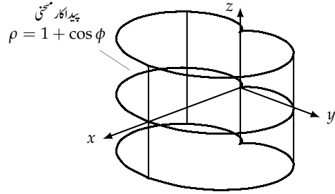
شکل ۱۱.۶۴: قلب نما مساوات \rho = 1 + \cos \phi فضائیں نکلی کو ظاہر کرتی ہے جس کی عمودی تراش محور z کو قائمہ ہے (مثال ۱۱.۵۶)۔
