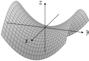
شکل ۱۳.۶۱: مبداء اس تعامل کا نقطہ زین ہے۔ اس تعامل کے کوئی بھی مقامی انتہائی قیمتیں موجود نہیں ہیں۔
