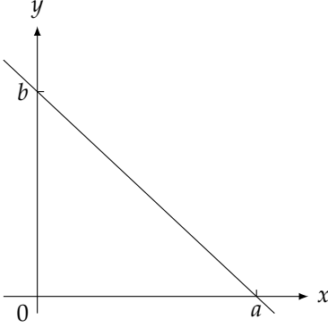
شکل ۱.۱۲: غیر انتصابی اور غیر افقی خط کے محوری قطعات
