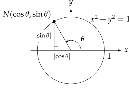
شکل ۱.۶۵: عمومی زاویہ \theta کے لیے حوالہ مکون۔
