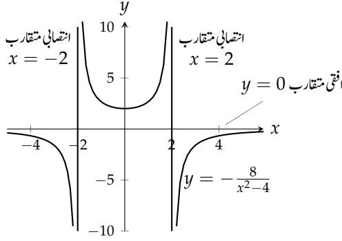
شکل ۴.۶۷: انتصابی مقارب (مثال ۴.۲۸)
