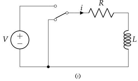
شکل ۶۸. ۷: سلسلہ دار مزاحمت و امالہ برقی دور (مثال ۸۹. ۷)
