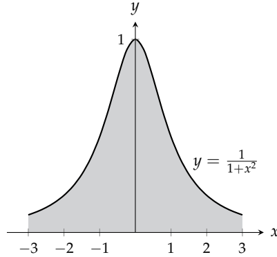
شکل ۸.۲۲: دونوں اطراف لامتناہی منحنی کے نیچے رقبہ متناہی ہے۔
