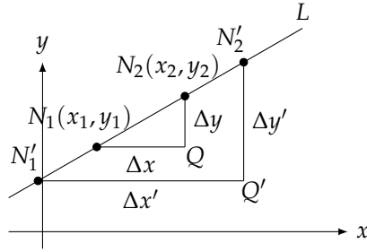
شکل ۱.۷: N_1'Q'N_2' اور N_1QN_2 متشابہ مثلثات ہیں لہذا \frac{\Delta y}{\Delta x} = \frac{\Delta y'}{\Delta x'} ہوگا
