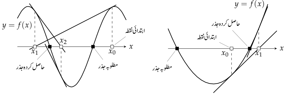
شکل ۱۰۳: ترکیب نیوٹن کسی دوسرے جذر پر مرکوز ہو سکتا ہے۔
