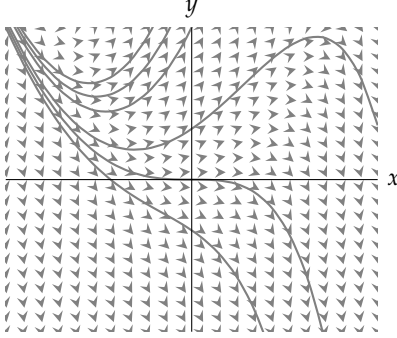
(ب) میدان ڈھلوان پر مخصوص منحنيات حل۔
