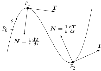
شکل ۱۲.۲۰: مخفی کا عمودی سمتیہ \frac{dT}{ds} ہر وقت اس رخ ہوتا ہے جس رخ T مڑتا ہو۔ سمتیہ N کا رخ سمتیہ \frac{dT}{ds} کا رخ ہے۔
