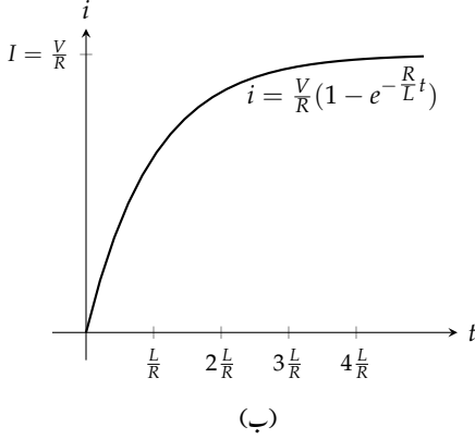
شکل ۶۸. ۷: سلسلہ وار مزاحمت و امالہ برقی دور (مثال ۸۹. ۷)
