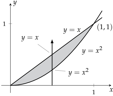
شکل ۱۶.۱۶: قطعہ مکانی اور لکیر کے رقبہ (مثال ۱۴.۵)۔
