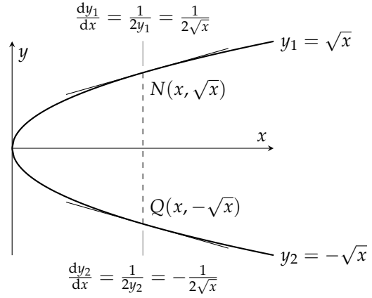
شکل ۳.۵۵: ترسیم برائے مثال ۳.۴
