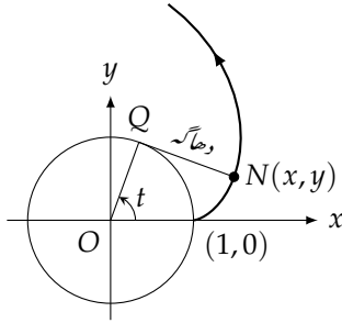
شکل ۱۰.۴۵: اکائی دائرے کا درپچیدہ (سوال ۳۰)
