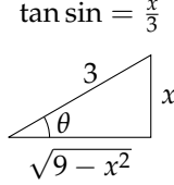
شکل ۸.۱۱: حوالہ مثلث برائے مثال ۲
