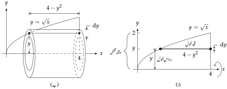
شکل ۶.۱۰: محور x کے گرد طواف (مثال ۲)
