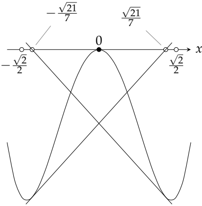
شکل ۴.۱۰۵: ترکیب نیوٹن ابتری کا شکار ہے۔
