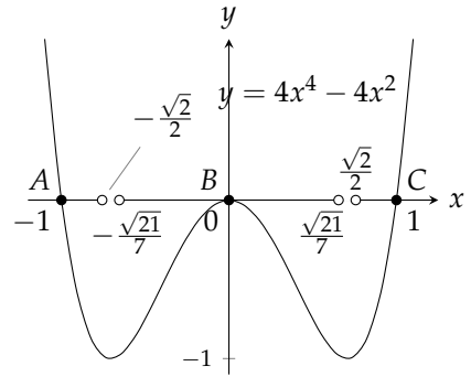
شکل ۴.۱۰۵: ترکیب نیوٹن ابتری کا شکار ہے۔
