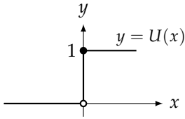
شکل ۲.۵۹: یہ تفاعل مبداء دائیں استمراری ہے
