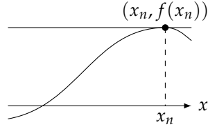
شکل ۴.۱.۲: اگر f'(x_n) = 0 ہو تب نقطہ قطع نہیں پایا جاتا ہے لہذا ترکیب نیوٹن رک جاتی ہے اور x_{n+1} ناقابل معلوم ہو گا۔
