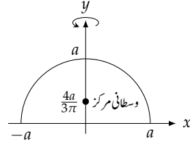
شکل ۶.۱۴: نصف کرہ کا وسطانی مرکز (مثال ۶.۴۳)
