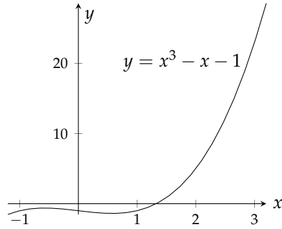
شکل ۴.۹۸: منحنی f(x) = x^3 - x - 1 کو محور x کے قریب سے قطع کرتی ہے۔
