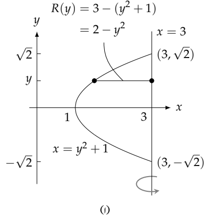
شکل ۱.۶.۳: مستوی خط اور جسم طواف (مثال ۱.۶.۱۲)
