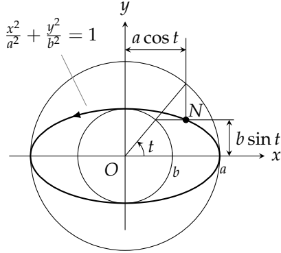
شکل ۱۰.۳۹: تریخیمی راہ (مثال ۱۰.۱۷)
