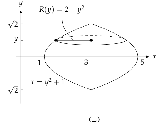
شکل ۱.۶.۳: مستوی خط اور جسم طواف (مثال ۱.۶.۱۲)
