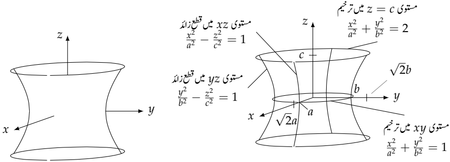
شکل ۱۱.۵: ایک چادری قطع زائد سطح
