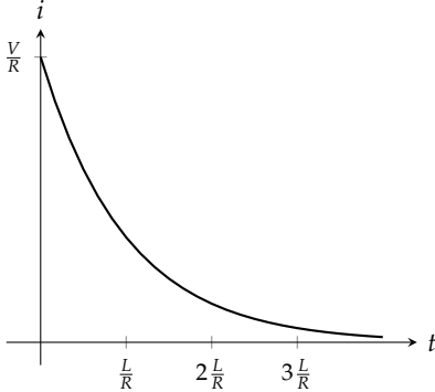
شکل ۷.۷۰: تنزل برقی رو (سوال ۷.۷۴)
