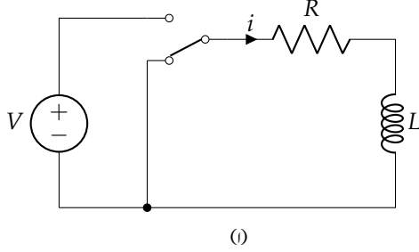
شکل ۷.۷: سلسلہ وار مزاحمت، امالہ برقی دور (مثال ۷.۹)
