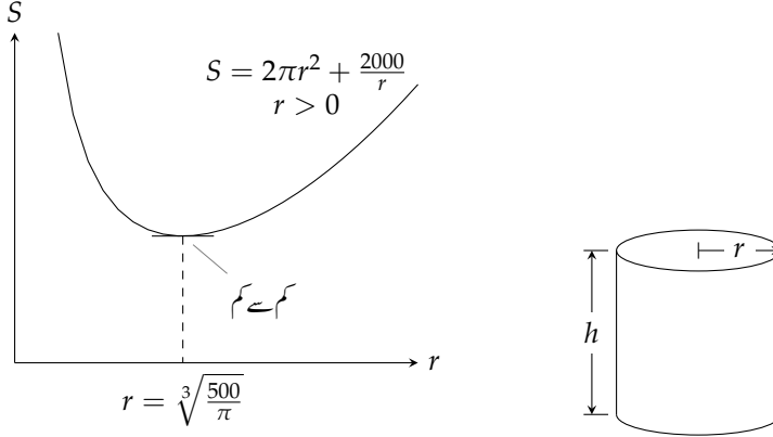
شکل ۴.۱۱۱: ٹین کا ڈبہ (مثال ۴.۲)
