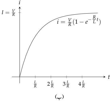
شکل ۷.۷: سلسلہ وار مزاحمت، امالہ برقی دور (مثال ۷.۹)
