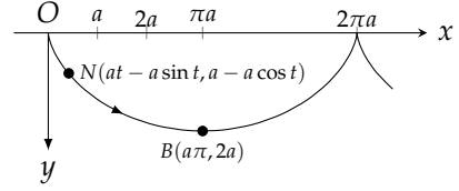
شکل ۱۰.۴۲: سر نیچے تدویر پر کشش ثقل کی بنا حرکت۔
