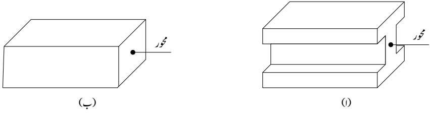
شکل ۱۴.۱۹: دونوں شہتیر کا رقبہ عمودی تراش ایک جیسا ہے لیکن شہتیر-اکا جمودی معیار اثر زیادہ ہے لہذا شہتیر-از زیادہ اکڑ ہو گا۔
