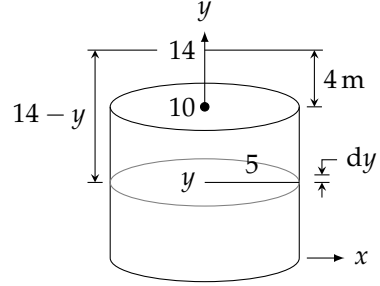
شکل ۶.۱۱۴: بیلنی حوض (مثال ۶.۶)
