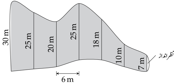
شکل ۵.۳: گندے پانی کا تالاب۔ افقی فاصلے 6 m ہیں (مثال ۵.۶)۔
