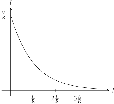
شکل ۷.۷: تنزل برقی رو (سوال ۷.۵۲)
