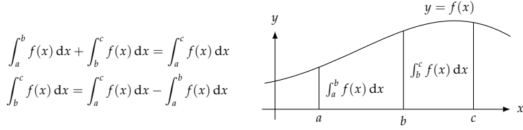
شکل ۵.۴: قطعی مکمل کی جمع پذیری
