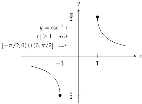
شکل ۷.۴۸: y = \csc^{-1} x ترسیم
