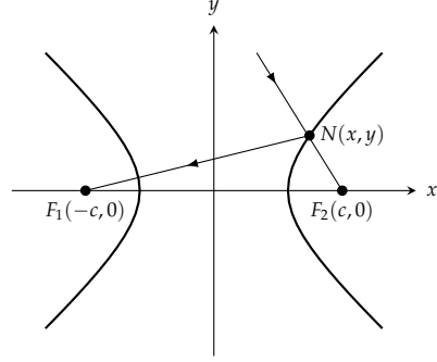
شکل ۱۰.۳۵: قطع زائد برائے سوال ۱۰.۳۱
