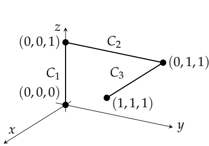
شکل ۱۵.۱۴: ٹکڑوں میں خطی راہ برائے سوال ۱۵.۱۶
