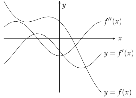
شکل ۴.۴.۴: تقابل y = f(x) = 2 \cos x - \sqrt{2}x اور اس کے یک رتہی اور دور تہی تفرقی۔
