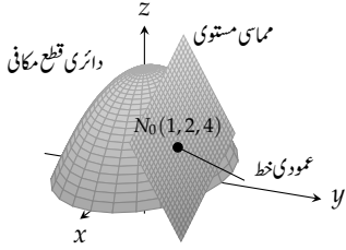
شکل ۱۳.۵۰: نقطہ N_0 پر دائری قطع مکانی سطح کا مماسی مستوی اور عمودی خط (مثال ۱۳.۶)۔
