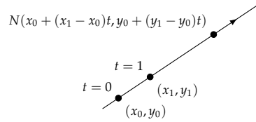
شکل ۱۰.۴۷: مستوی میں سیدھی لکیر (سوال ۱۰.۳۱)
