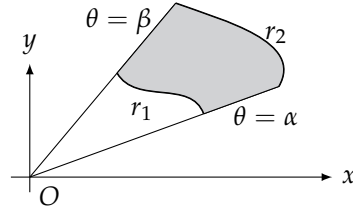
شکل ۱۰.۱۳۹: سایہ دار رقبہ تلاش کرنے کی خاطر r_2 اور مبدا کے رقبہ سے r_1 اور مبدا O کے رقبہ منہی کیا جاتا ہے۔
