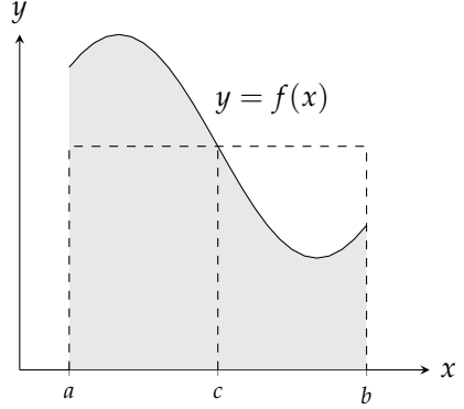
شکل ۵.۵: وقفہ [a, b] کے کسی نقطہ c پر \int_a^b f(x) dx = f(c) \cdot (b - a) ہوگا۔
