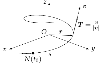
شکل ۱۲.۱۳: ہم v کو |v| سے تقسیم کر کے مماسی اکائی سمتیہ T حاصل کرتے ہیں۔
