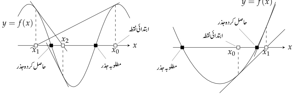
شکل ۱۴.۱۳۲: ترکیب نیوٹن کسی دوسرے جذر پر مرکوز ہو سکتا ہے۔
