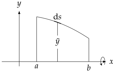
شکل ۲.۱۳۴: مسئلہ پاپس برائے سطحی رقبہ (مسئلہ ۲.۲)
