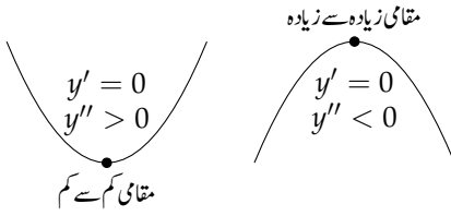
شکل ۴.۴.۴: دور تہی تفرقی پرکھ برائے مقامی انتہا
