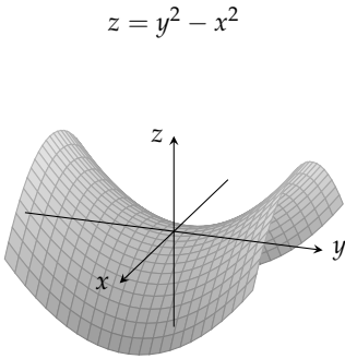
شکل ۱۳.۶۱: مبدا اس تقابل کا نقطہ زین ہے۔ اس تقابل کے کوئی بھی مقامی انتہائی قیمتیں موجود نہیں ہیں۔
