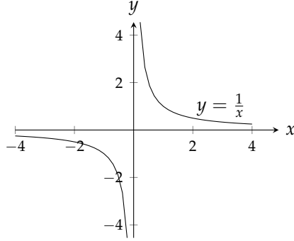
شکل ۴.۴۳: تفاعل y = \frac{1}{x} کی ترسیم۔
