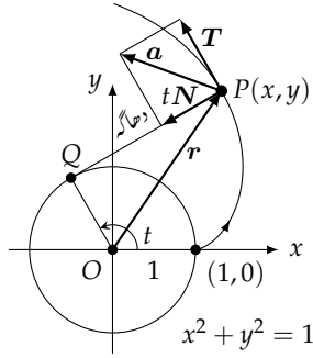
شکل ۱۲.۲: اسراع کے مماسی اور عمودی اجزاء (مثال ۱۲.۶)
