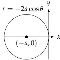
شکل ۱۰.۱۴: کار تیمی محور پر مرکز والے دائروں کے قطبی مساوات۔
