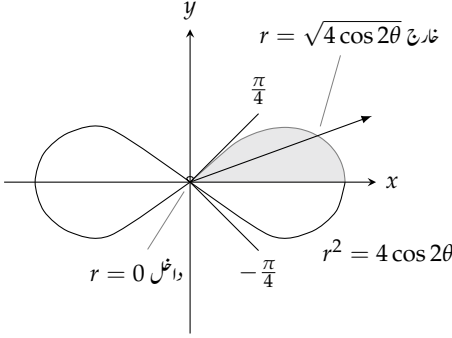
شکل ۱۴.۲: تکمل کی قیمت کے حصول میں ہم r کو 0 تا \sqrt{4 \cos 2\theta} جبکہ \theta کو 0 تا \pi/4 لیتے ہیں۔
