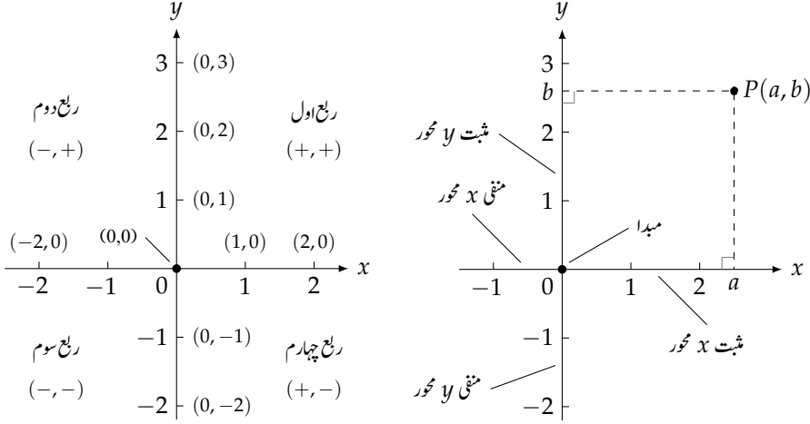
شکل ۱.۲: کارٹیزی محدد
