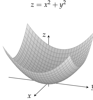
شکل ۱۳.۶۰: تقابل f(x, y) = x^2 + y^2 کی ترسیم قطع مکانی سطح z = x^2 + y^2 ہے۔ اس تقابل کا ایک فاصل نقطہ پایا جاتا ہے، جو مبدا پر ہے اور جس پر مقامی کم سے کم قیمت 0 پائی جاتی ہے۔
