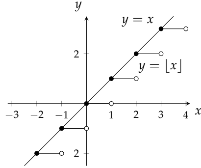
شکل ۱.۳: عدد صحیح زمین تفاعل (مثال ۱.۸)
