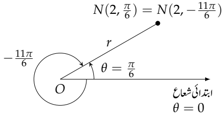
شکل ۱۰.۸۸: قطبی محدود دیکھتا نہیں ہیں۔
