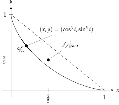
شکل ۱۰.۸۲: ستارہ نما کا وسطانی مرکز۔
