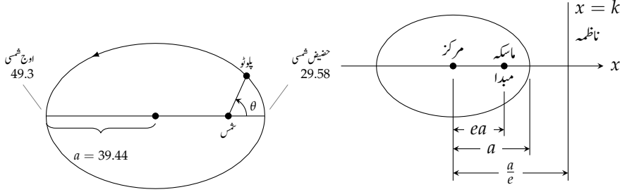
شکل ۱۰.۱۲۸: مدار پلوٹو (مثال ۱۰.۶)
