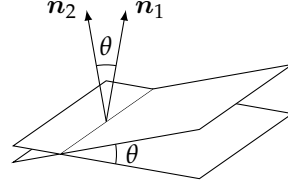
شکل ۱۱.۶۳: دو سطحوں کے تقاطع زاویہ، ان سطحوں کے عمودی سمتیات کے تقاطع زاویہ کے برابر ہوتا ہے۔
