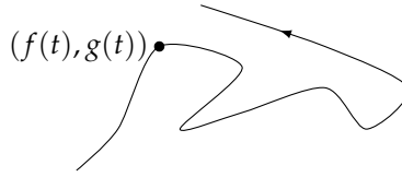
شکل ۱۰.۵۳: مستوی xy میں ضروری نہیں کہ ذرے کی راہ x یا y کا تقابل ہو۔
