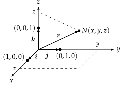
شکل ۱۱.۳۱: فضا میں نقطے کا تعین کر سمتیہ۔
