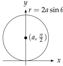
شکل ۱۰.۱۴: کار تیمی محور پر مرکز والے دائروں کے قطبی مساوات۔
