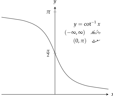
شکل ۸.۴۶: ترسیم y = \cot^{-1} x
