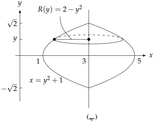
شکل ۶.۲۳: مستوی خطہ اور جسم طواف (مثال ۶.۲)
