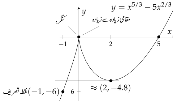
شکل ۴.۵۰: تقابل y = x^{5/3} - 5x^{2/3} کی ترسیم (مثال ۴.۷)
