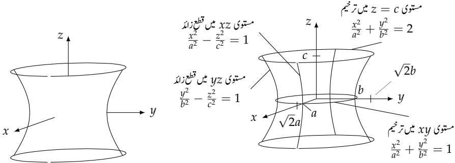
شکل ۱۱.۷۳: ایک چادری قطع زائد سطح
