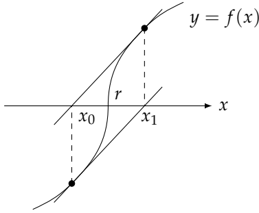
شکل ۴.۱۴: ترکیب نیوٹن کی عدم مرکزیت۔
