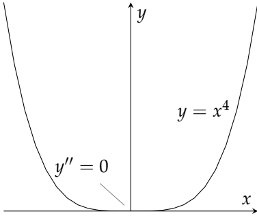
شکل ۴.۴۲: اگرچہ مبدأ پر y'' = 0 ہے یہاں نقطہ تعریف نہیں پایا جاتا ہے (مثال ۴.۵)
