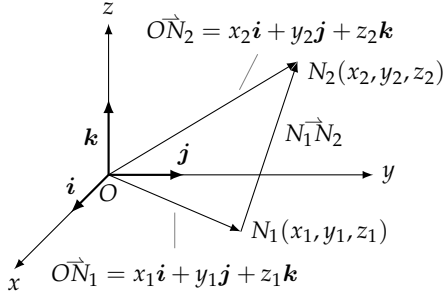
شکل ۱۱.۳۲: دو نقطوں کے بیچ سمتیہ۔
