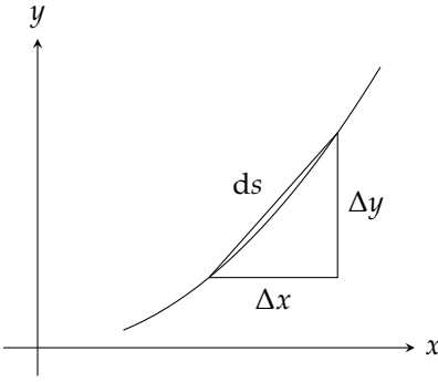
شکل ۶.۷۸: تعلق ds = \sqrt{dx^2 + dy^2} کا حصول۔
