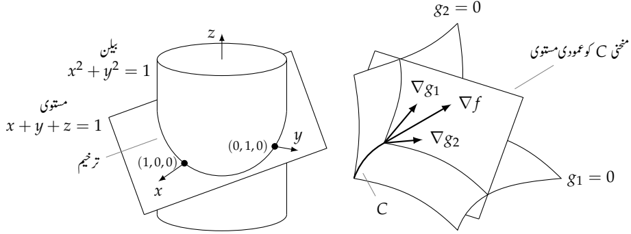
شکل ۱۳.۴۲: جس ترخیم پر بیلن اور مستوی ایک دوسرے کو قطع کرتے ہیں اس پر مبداسے دور تر اور نزدیک تر نقاط کی تلاش۔
