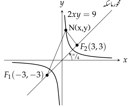
شکل ۱۰.۳۹: قطع زائد 2xy = 9 کا محور ماسک، مثبت x محور کے ساتھ \frac{\pi}{4} زاویہ بناتا ہے۔
