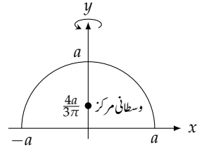
شکل ۲.۱۳۳: نصف کرہ کا وسطانی مرکز (مثال ۲.۳)
