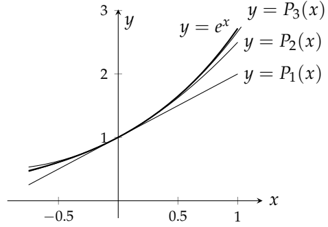
شکل ۹.۲۶: قوت نمائی تفاعل f(x) = e^x کی ٹیلر کثیر رکنیاں (مثال ۹.۲)
