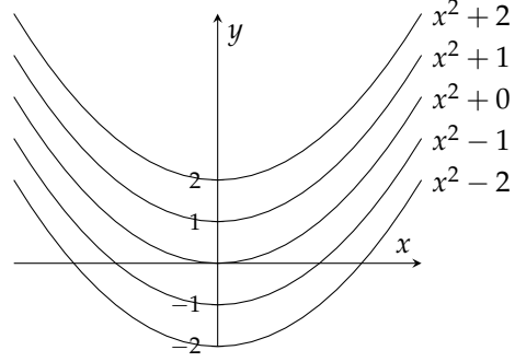
شکل ۴.۲۱: ضمنی نتیجہ ۴.۲ کہتا ہے کہ ایک جیسے تفرق والے تفاعل میں صرف انتظامی فرق پایا جاتا ہے۔
