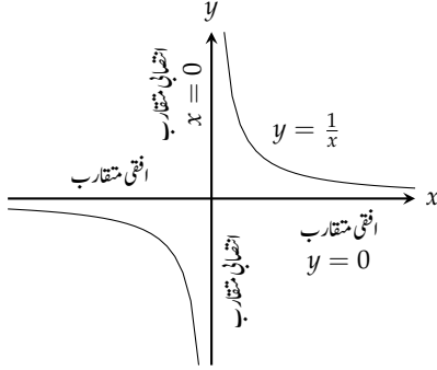
شکل ۴.۸: محدوی محور قطع زائد y = \frac{1}{x} کے دونوں شاخوں کے متقارب ہیں۔
