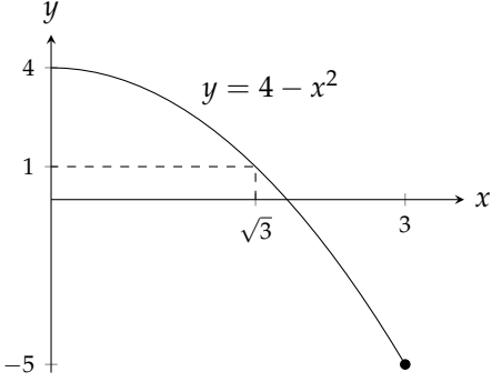
شکل ۵.۴۵: وقفہ [0, 3] پر تفاعل f = 4 - x^2 کی اوسط قیمت 1 کو تفاعل x = \sqrt{3} پر اختیار کرتا ہے (مثال ۵.۷)۔
