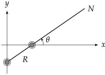
شکل ۱۰.۴۸: آرشمیدی روک برائے سوال ۱۰.۳۲
