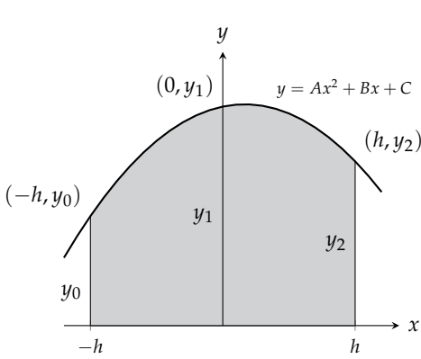
شکل ۵.۴۲: سایہ دار رقبہ \frac{h}{3}(y_0 + 4y_1 + y_2) ہے۔
