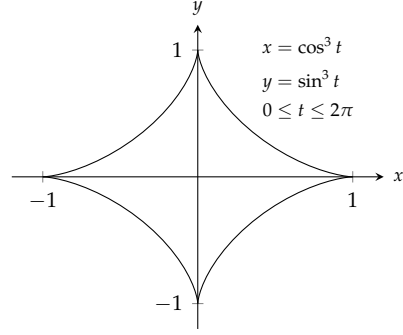
شکل ۱۰.۸۳: ستارہ نما برائے مثال ۱۰.۳
