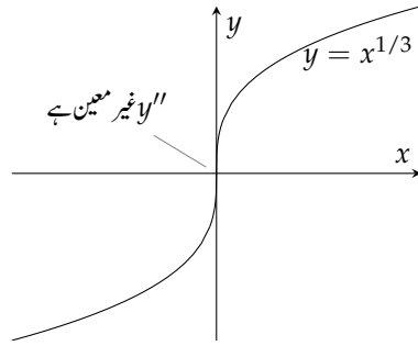
شکل ۴.۴۴: نقطہ تعریف پر y'' غیر معین ہے (مثال ۴.۴)
