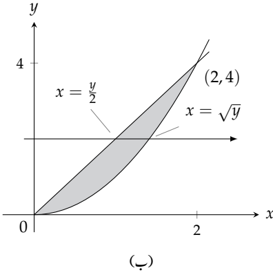
شکل ۱۴.۲: دو منحنیات کے بیچ خطہ (مثال ۱۴.۴)
