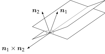
شکل ۱۱.۶۴: سطحوں کا خط تقاطع کا سطحوں کے عمودی سمتیات کے ساتھ تعلق۔
