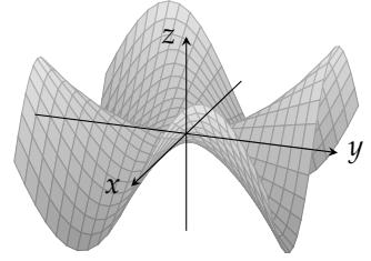
شکل ۵۷: z = \frac{xy(x^2 - y^2)}{x^2 + y^2}
