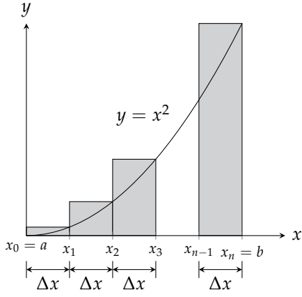
شکل ۵.۳۴: ریمان مجموعوں کے مستطیل (مثال ۵.۹)
