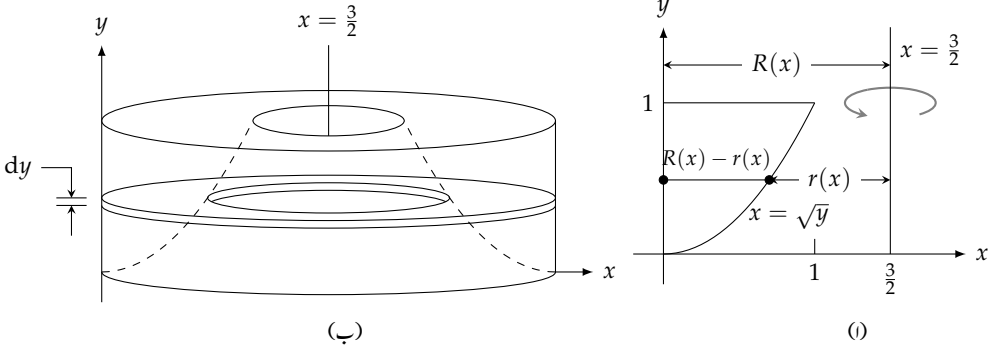
شکل ۶.۴: جسم طواف اور نمائندہ چھلا (مثال ۶.۷)
