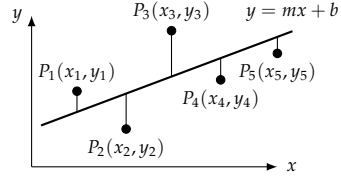
شکل ۱۳.۶۴: غیر ہم خطی نقاط پر سیدھا خط بٹھانے کے لئے ہم وہ کلیئر منتخب کرتے ہیں جس میں انتہائی فرق کے مربع کا مجموعہ کم سے کم ہو۔
