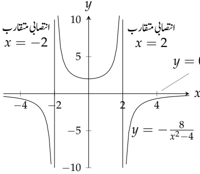
شکل ۴.۸۲: انتصابی مقارب (مثال ۴.۹)
