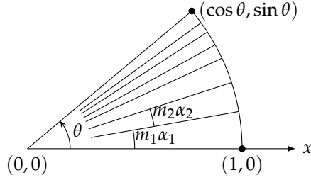
شکل ۱۰.۵: سائن اور کوسائن حاصل کرنے کا عمل۔
