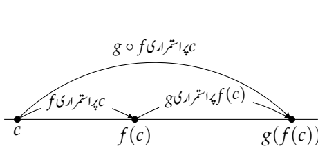
شکل ۲.۶۷: مرکب تفاعل کی استمرار۔
