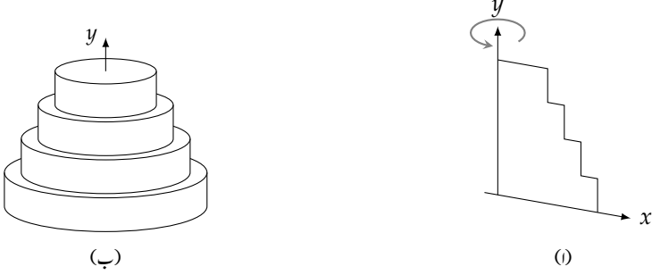
شکل ۶.۵: تکلی جسم طواف
