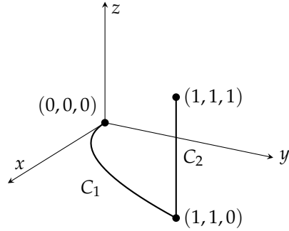
شکل ۱۵.۱۵: راہ برائے مکمل (سوال ۱۵.۱۵)
