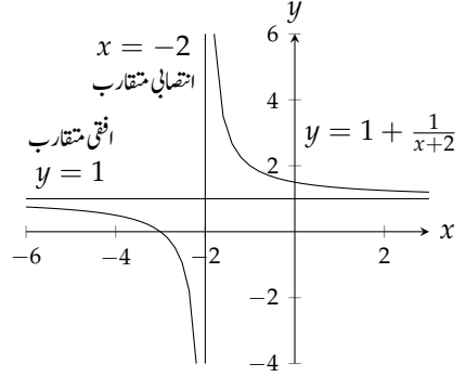
شکل ۴.۸۱: انتصابی مقارب (مثال ۴.۸)
