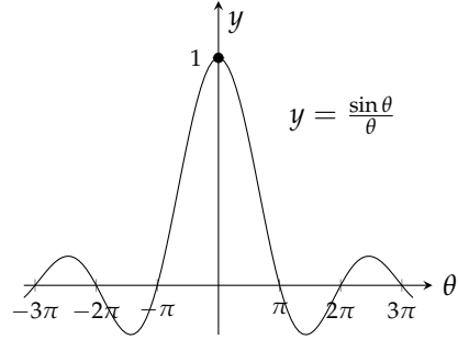
شکل ۳.۴۴: تقابل f(\theta) = \frac{\sin \theta}{\theta} جہاں \theta کی پیمائش ریڈین میں ہے۔
