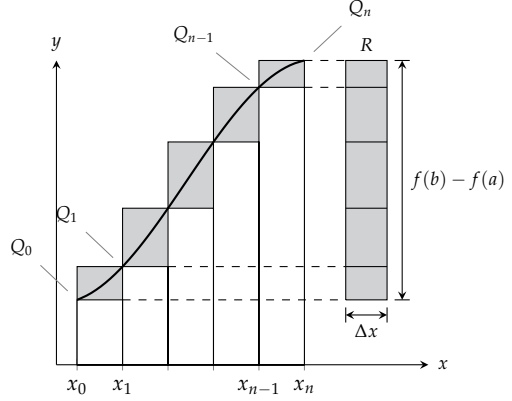
شکل ۵.۴۱: بالائی اور زیریں مجموعوں میں فرق [f(b) - f(a)]\Delta x ہوگا۔
