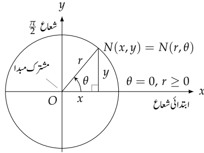
شکل ۱۰.۹۳: کار تیسہ اور قطبی محدود کے تعلقات معلوم کرنے کا عمومی طریقہ۔
