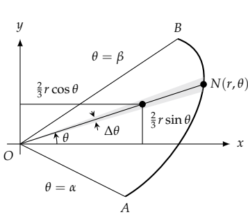
شکل ۱۰.۱۵۲: باریک سایہ دار خطے کے معیار اثر۔
