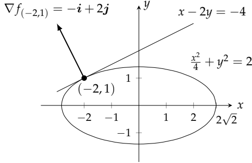
شکل ۱۳.۳۸: ہم قطع مکانی کو تقاطع f(x, y) = \frac{x^2}{4} + y^2 کی ہم قد منحنی تصور کر کے اس کا مماس تلاش کر سکتے ہیں (مثال ۱۳.۳۳)۔
