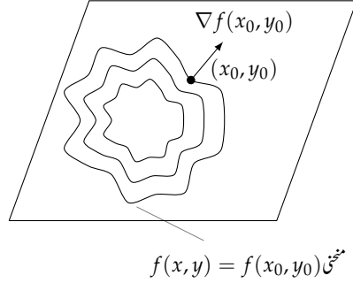
شکل ۱۳.۳۹: دو متغیرات کے تقاطع کی ڈھلوان ہر صورت ہم قد منحنیات کی عمودی ہوگی۔
