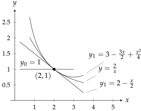
شکل ۹.۲۴: تقاع f(x) = \frac{2}{x} اور اس کی ابتدائی تین تخمینی کثیر رکنیاں (مثال ۹.۴۸)۔
