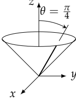
شکل ۱۱.۶۹: ترخیم برائے مثال ۱۱.۶۱
