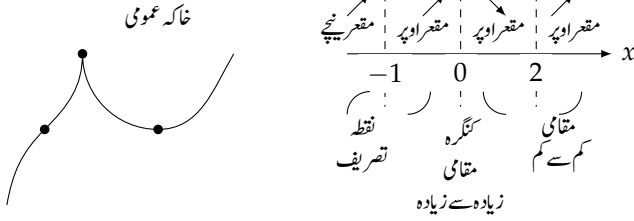
شکل ۴.۴۵: ۱: جمال اور خاکہ کے (مثال ۴.۱۹)
