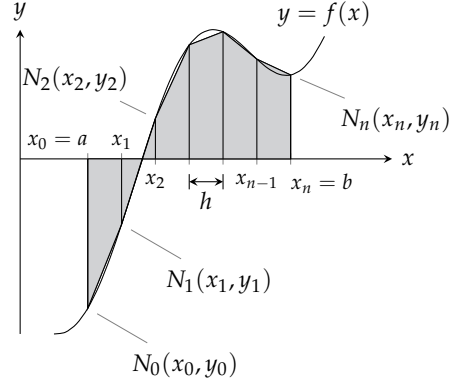
شکل ۵.۹۲: ذوزنقہ قاعدہ برائے عددی مکمل۔
