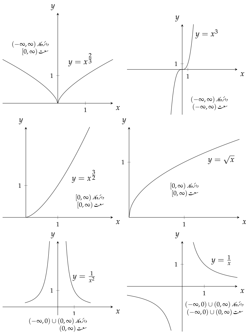
شکل ۱.۲۱: چند اہم تفاعل کی ترسیم
