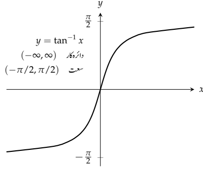
شکل ۱.۳۹: y = \tan^{-1} x ترسیم
