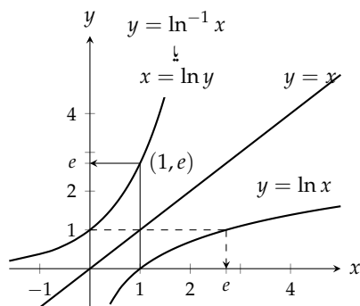
شکل ۱.۲۶: تفاعل y \ln x اور تفاعل y = \ln^{-1} x - عدد e سے مراد \ln^{-1} 1 ہے۔
