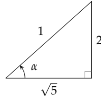
شکل ۱.۳۴: مثلث کی مدد سے زاویوں کا حصول (مثال ۱.۵)
