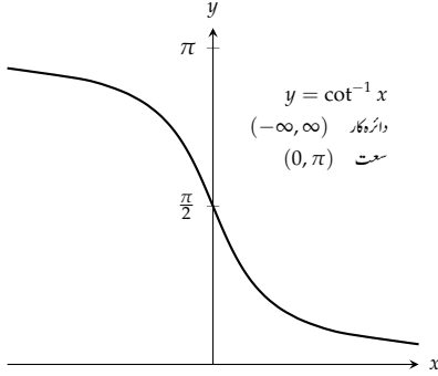
شکل ۱.۴۰: y = \cot^{-1} x ترسیم
