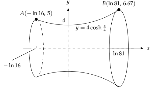
شکل ۱.۲۴: مکر سطح (سوال ۱.۲۹)
