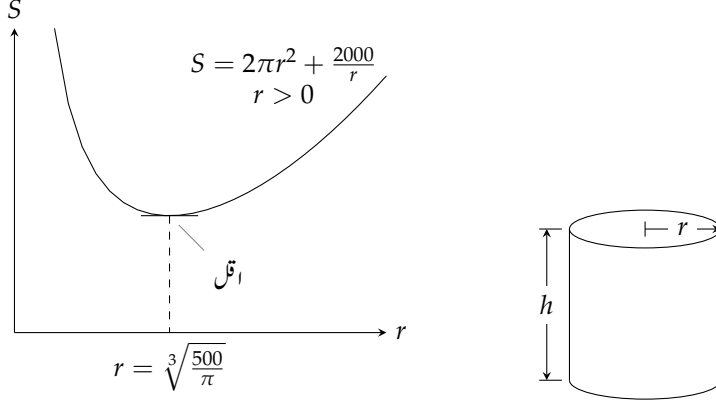
شکل ۷.۳: ٹین کا ڈبہ (مثال ۴.۳۴)
