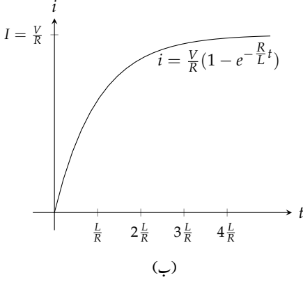
شکل ۷.۷۲: سلسلہ وار مزاحمت، امالہ برقی دور (مثال ۷.۸۳)
