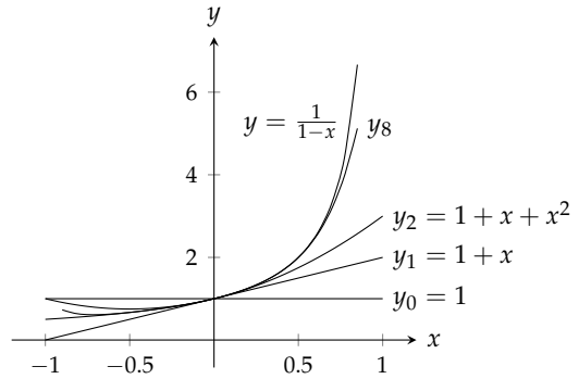
شکل ۹.۲۳: تقابل f(x) = \frac{1}{1-x} اور اس کی چار تخمینی کثیر رکنیاں (مثال ۹.۲۷)۔
