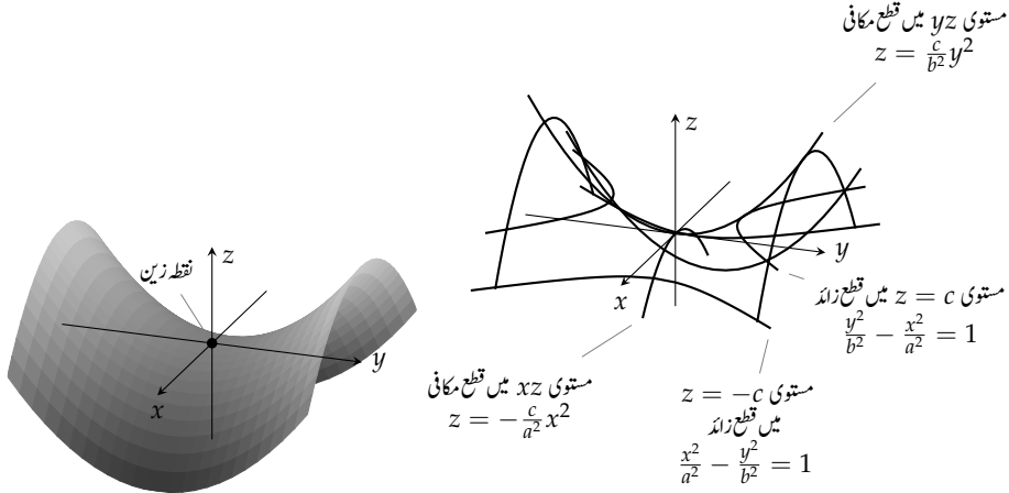
شکل ۱۱.۷۵: قطع زائد قطع مکانی سطح
