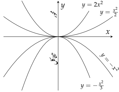
شکل ۱.۴.۷: قطع مکانی y = ax^2
