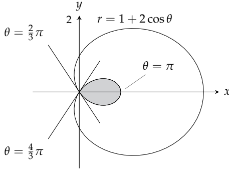
شکل ۱۰.۱۳۶: رقبہ گھونگا (مثال ۱۰.۱۳۶)
