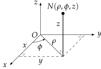
شکل ۱۱.۷: فضائیں نقطہ کے تکلی محدود \rho ، \phi اور z ہوں گے۔
