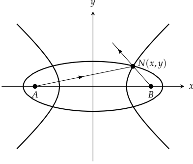
شکل ۱۰.۳۶: قطع زائد اور ترخیم برائے سوال ۱۰.۱۳۲
