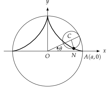
شکل ۱۰.۴۹: ستارہ نما۔ سوال ۱۰.۲۱۴
