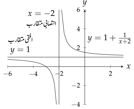
شکل ۴.۸۱: انتصابی مقارب (مثال ۴.۲۷)
