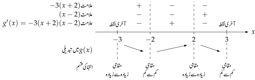
شکل ۴.۳۴: تفرق کی علامتوں سے تفاعل کا رویہ (مثال ۴.۱۲)
