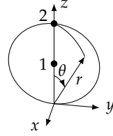
شکل ۱۱.۸۳: کرہ برائے مثال ۱۱.۶۰
