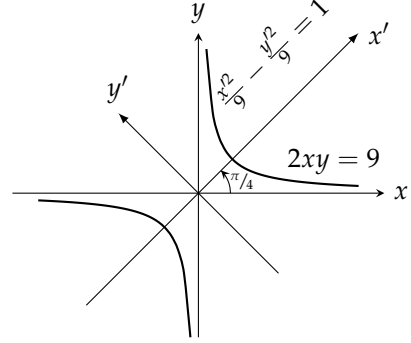
شکل ۱۰.۴۹: نئے محور x' اور y' میں قطع زائد کی مساوات (مثال ۱۰.۱۰)
