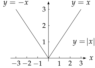
شکل ۲.۶۶: تفاعل کا کونا اس کو استراری ہونے سے نہیں روکتا ہے (مثال ۲.۳۴)۔
