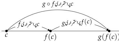
شکل ۲.۶۷: مرکب تفاعل کی استرار۔
