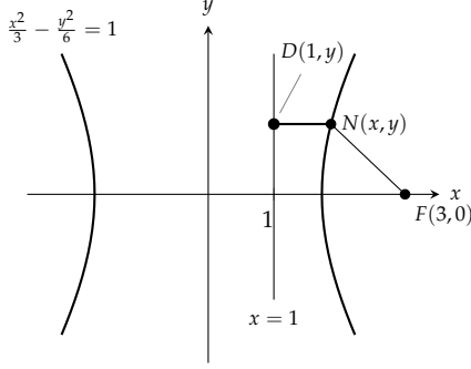
شکل ۱۰.۴۳: قطع زائد برائے مثال ۱۰.۹
