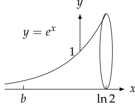
شکل ۸.۲۱: ٹھوس نگل کا حجم (مثال ۸.۴۲)
