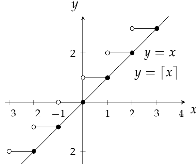
شکل ۱.۲۷: عدد صحیح چھت تقاض (مثال ۱.۲۹)
