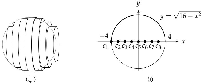
شکل ۵.۱۹: نصف دائرہ y = \sqrt{16 - x^2} کو x محور کے گرد گما کر کرہ حاصل کیا جاتا ہے (مثال ۵.۲۴)۔
