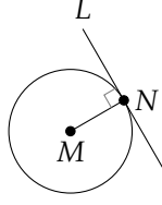
شکل ۲.۴۵: نقطہ N پر مماس اور رداس آپس میں عمودی ہیں۔
