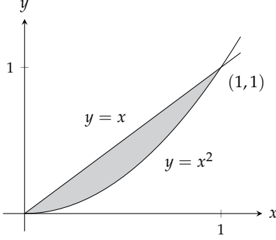
شکل ۱۴.۹: خطہ برائے مثال ۱۴.۹
