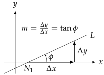
شکل ۱.۱۰: غیر انتصابی خط کی ڈھلوان اس کے زاویہ میلان کا ٹینجینٹ ہوتا ہے
