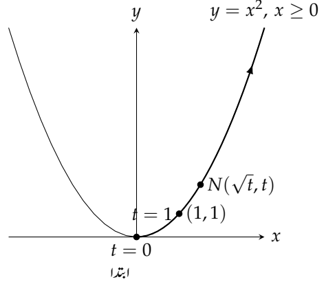
شکل ۱۰.۵۶: نصف قطع مکانی راہ (مثال ۱۰.۱۵)
