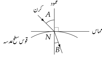
شکل ۳.۵۹: عرصہ میں کرن داخل ہوتے ہوئے عمود کی طرف جھکتی ہے۔
