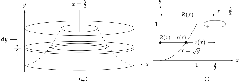
شکل ۶.۴: جسم طواف اور نمائندہ چھلا (مثال ۶.۱۵)
