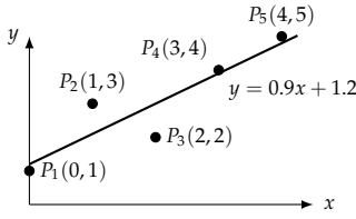
شکل ۱۳.۶۵: کمترین مربعات خط۔
