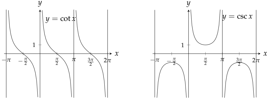
شکل ۴.۸۰: انتظامی مقارب (مثال ۴.۲۶)
