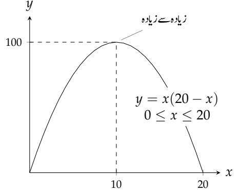
شکل ۴.۱۱۴: x اور (20 - x) کے حاصل ضرب کی زیادہ سے زیادہ قیمت 100 ہے (مثال ۴.۳۵)۔
