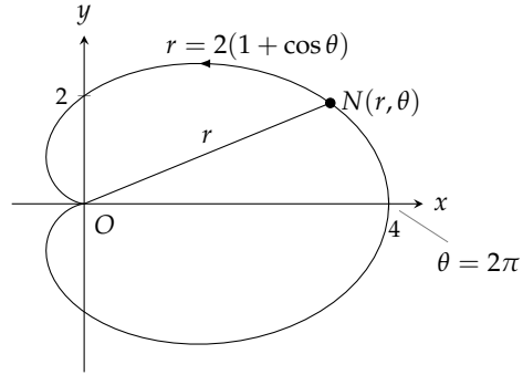
شکل ۱۰.۱۳۵: قلب نما کی ترسیم برائے مثال ۱۰.۱۳۵
