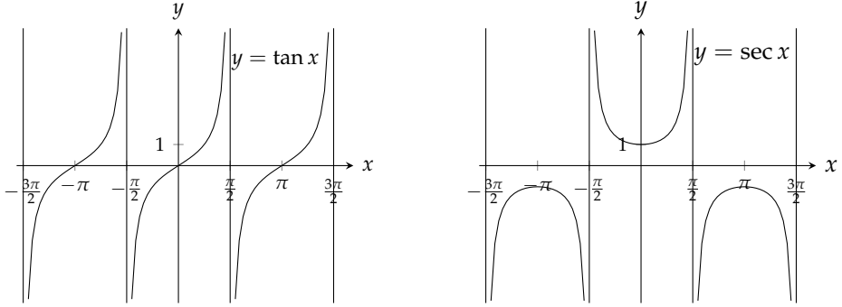
شکل ۴.۷۹: انتصابی مقارب (مثال ۴.۲۶)
