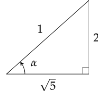
شکل ۵۰: مثلث کی مدد سے زاویوں کا حصول (مثال ۷.۵۷)
