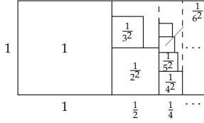
شکل ۹.۱۹: رقبوں کا مجموعہ 2 سے کم ہے (سوال ۹.۲۳۰)
