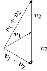
شکل ۱۱.۴۲: سمتیات برائے سوال ۱۱.۱۳۷۔
