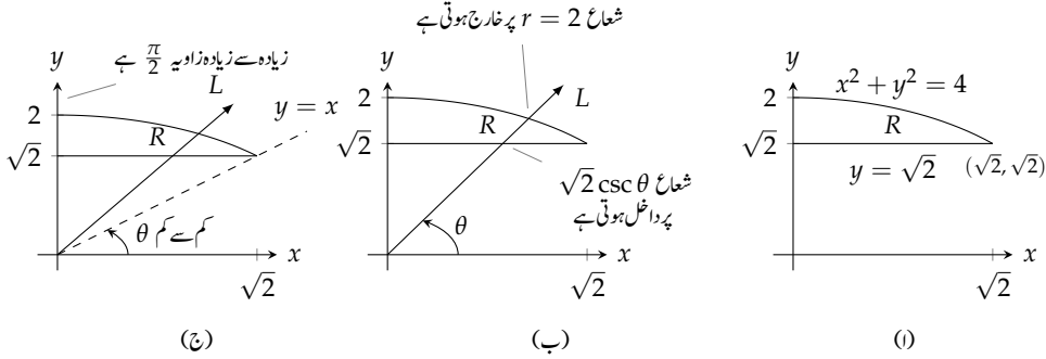
شکل ۱۴.۲۵: قطبی حدود میں تکامل کی قیمت کے قدم۔
