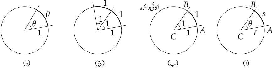
شکل ۱.۸۶: ریڈیئن کی تعریف
