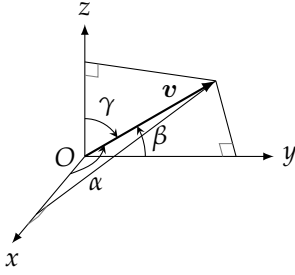
شکل ۱۱.۴۴: زاویات رخ اور کوسائن رخ کی تعریف برائے سوال ۱۱.۱۴۴۔
