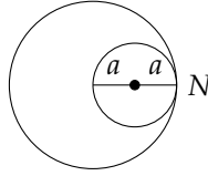
شکل ۱۰.۸۰: تدویر برائے سوال ۱۰.۲۱۵
