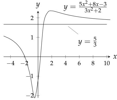
شکل ۴.۸: ترسیم تقابل اور حد (مثال ۴.۲۲)
