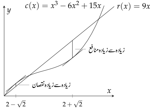
شکل ۴.۱۱۶: لاگت بالقابل منافع (مثال ۴.۳۸)
