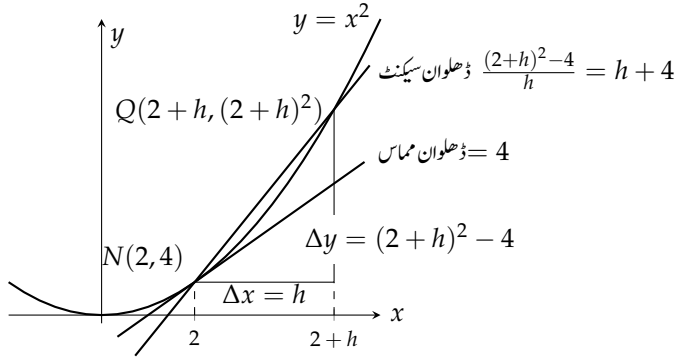
شکل ۲.۷: قطعہ مکانی کا مماس (مثال ۲.۳۹)
