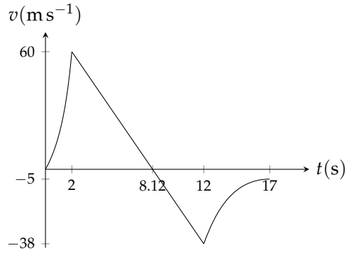
شکل ۳.۴۰: راکٹ کی حرکت (سوال ۱۳۹، ۳)
