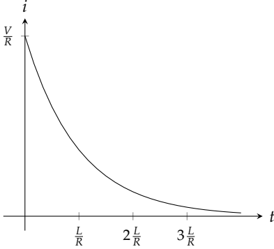
شکل ۷.۷۴: تنزل برقی رد (سوال ۷.۷۵)
