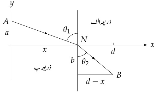
شکل ۱۱۴: ایک ذریعہ سے دوسرے ذریعہ میں داخل ہوتے ہوئے شعاع کی راہ (مثال ۳.۳)
