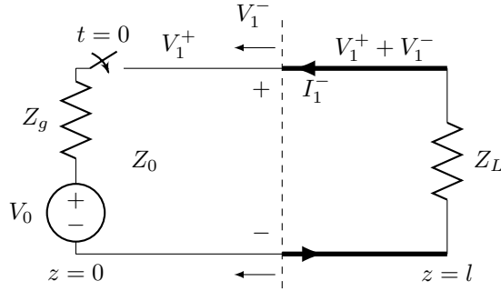
شکل ۱۱.۸: عمومی برقی بوجھ سے لدے ترسیلی تار میں ابتدائی موج۔
