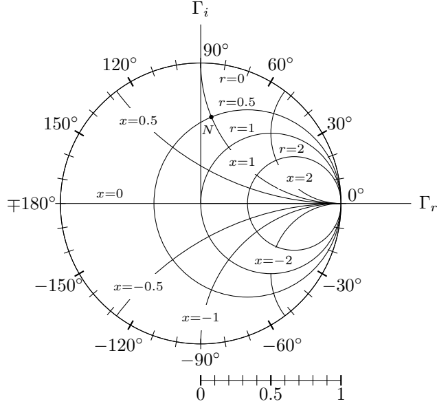
شکل ۱۱.۸: سمتھ نقشے پر اکائی دائرے میں r اور x سے حاصل دائرے دکھائے جاتے ہیں۔
