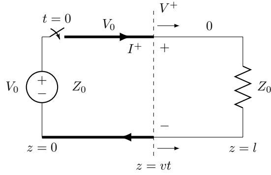
شکل ۱۱.۷: ترسیلی تار میں ابتدائی موج۔
