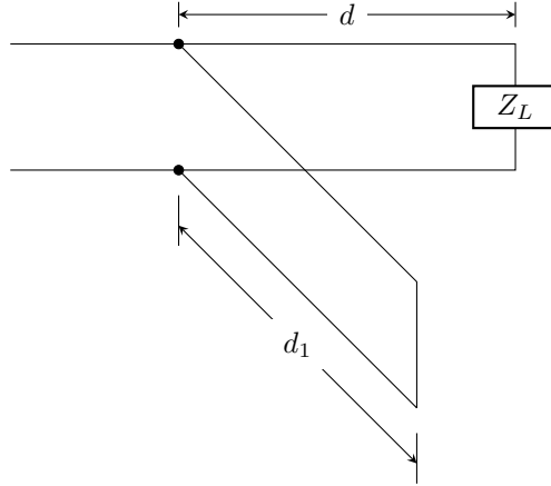
شکل ۱۱.۱۴: برقی بوجھ سے d فاصلے پر d_1 لمبائی کے قصر دور تار کا ککڑا جوڑنے سے برقی بوجھ اور ترسیلی تار ہمہ رکاوٹ بنائے جاتے ہیں۔
