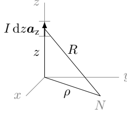
شکل ۷.۲۰: بتار کے چھوٹے حصے سے پیدا سمتی مقناطیسی دباؤ۔
