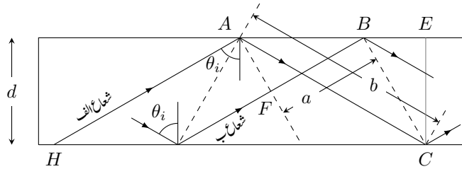
شکل ۱۳.۱۸: ذوبرق تختی کے اندرونی سطح پر ممکنہ آمدی زاویے۔
