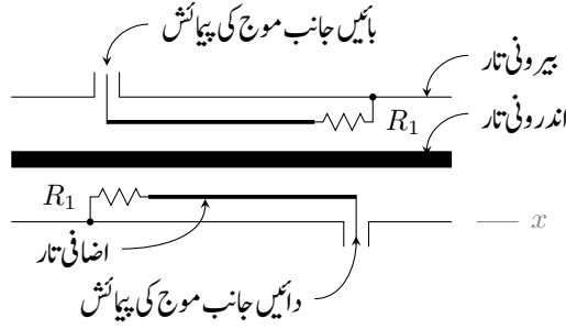
شکل ۱۱.۱۶: پیمائش سائین موج
