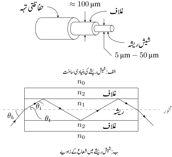
شکل ۱۳.۲۱: شیش ریشہ کی ساخت اور ممکنہ آمدی زاویے
