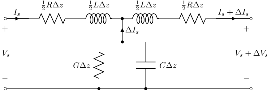
شکل ۱۱.۱: یکساں ترسیلی تار کا چھوٹا حصہ۔ متغیرات R, L, C, G تار کی شکل اور مادوں پر منحصر ہیں۔
