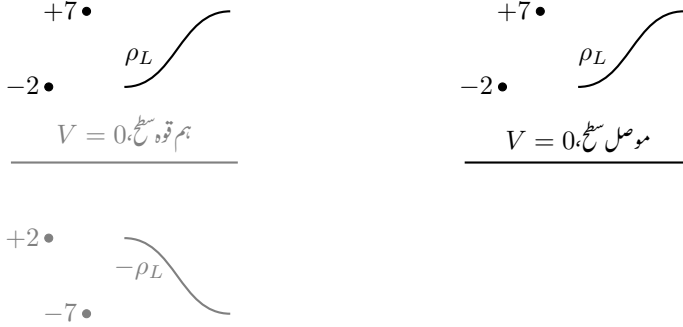
شکل ۵.۵: عکس کی ترکیب۔
