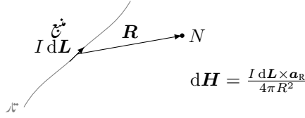
شکل ۱. ۷: بایوٹ سیوارٹ کا قانون۔
