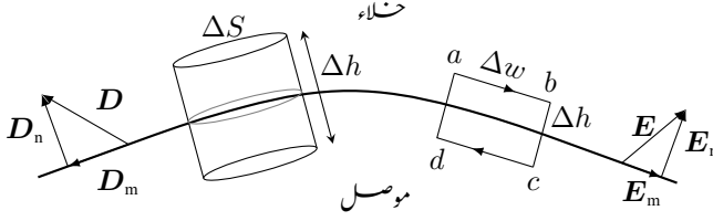
شکل ۵.۴: موصل اور خلاء کی سرحد پر برقی شرائط۔
