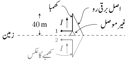
شکل ۱۴.۱۰: کھمبا اینٹینا
