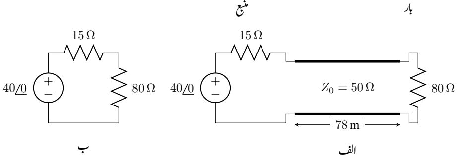
شکل ۱۱.۵: ترسیلی تار اور برقی بوجھ۔
