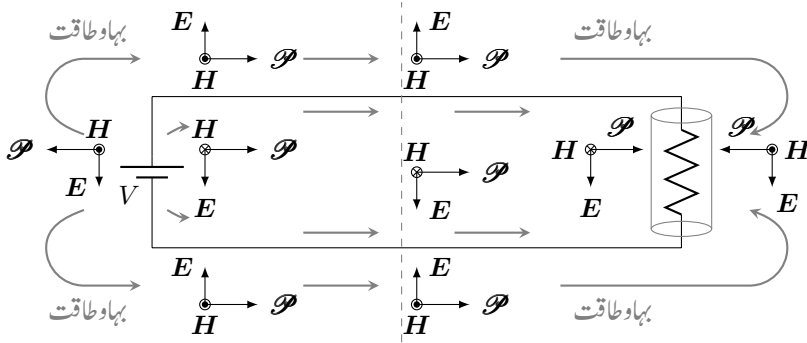
شکل ۱۰.۵: برقی دور میں طاقت کا بہاؤ۔
