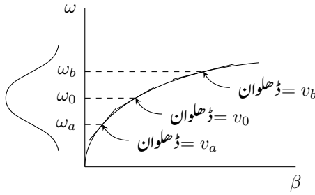
شکل ۱۲.۱۳: گوسی اشارے کا فوریز بدل تریلی ماڈے کے \beta - \omega خط پر دکھایا گیا ہے۔
