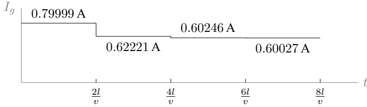
(ب) دیے نقطے کی برقی رد بالمتقابل وقت۔
