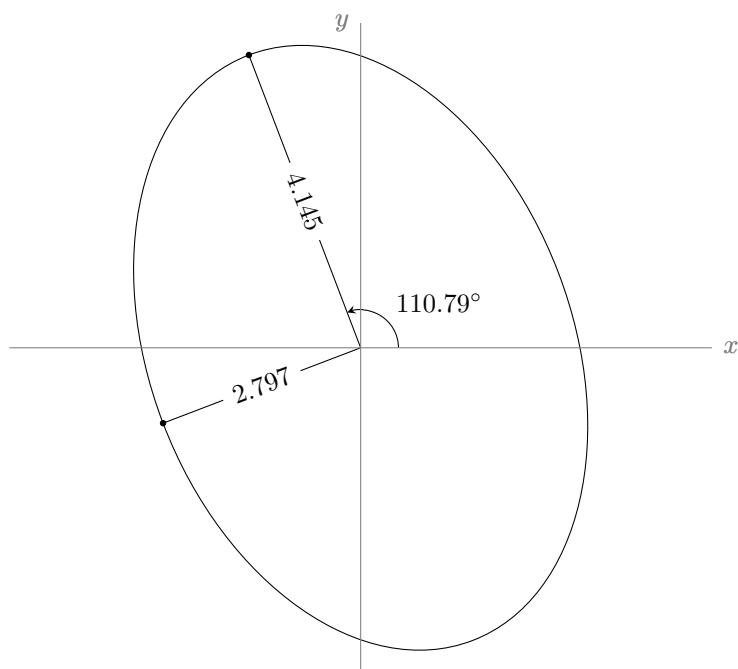
شکل ۱۰.۱۹: مثال ۱۰.۱۰ کی بیضوی قطبی موج۔
