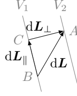
شکل ۴.۸: برقی دباؤ کی ڈھلوان برقی میدان ہے۔
