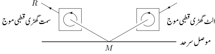
شکل ۱۲.۶: الٹ گھڑی قطبی آمدی موج موصل سطح سے انعکاس کے بعد سمت گھڑی قطبیت رکھتی ہے۔
