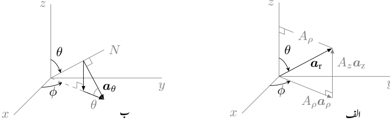
شکل ۱.۳۲: کروی اکائی سمتیات کا کارتیسی نظام میں تبادلو۔
