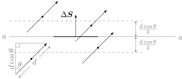
شکل ۵.۷: بیرونی میدان کی موجودگی میں مقید بار کی حرکت۔
