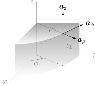
شکل ۱.۱۸: تکلی محدود کے اکائی سمتیات۔
