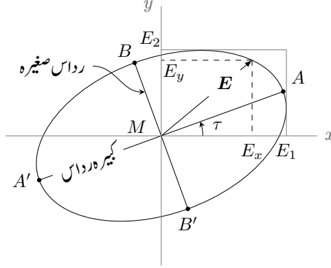
شکل ۱۰.۱۸: عمومی بیضی قطبیت۔
