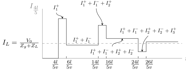
شکل ۱۱.۲۰: عارضی دورانی کی برقی رد و بالمتقابل برقی دباؤ۔
