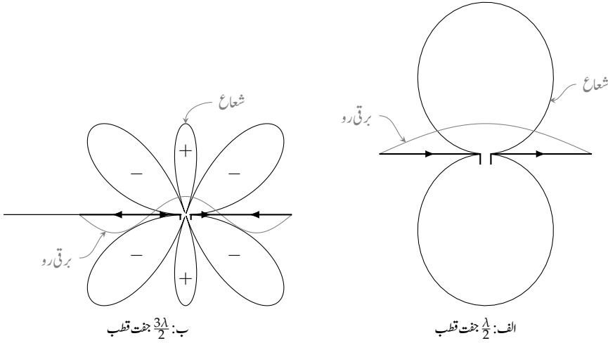
شکل ۱۴.۲۵: 0.5\lambda اور 1.5\lambda جفت قطب کے دو میدان۔
