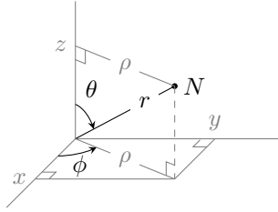
شکل ۱.۳۱: کروی، نکل اور کارتیسی متغیرات کا تبادلہ۔
