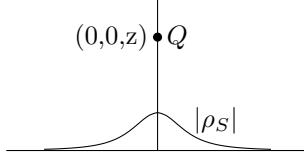
شکل ۵.۶: نقطہ بار سے لامحدود موصل سطح میں پیدا شدہ کثافت بار۔
