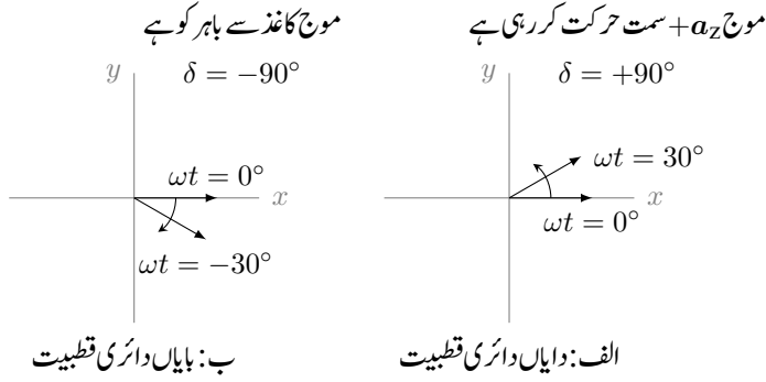
شکل ۱۰.۱: دائیں ہاتھ اور بائیں ہاتھ کی دائری قطبیت۔
