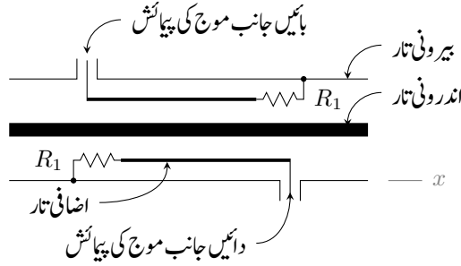
شکل ۱۱.۱۶: سمتی جوڑ گر
