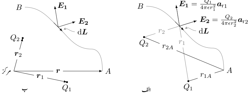
شکل ۳.۶: دو نقطہ بار کے میدان میں مطلق برقی دباؤ۔
