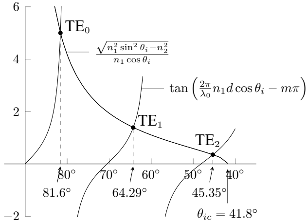
شکل ۱۹.۱۳: تغنی موج میں شعاع کے ممکن زاویے۔
