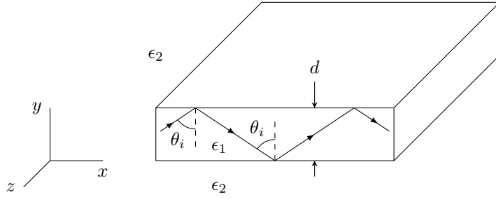
شکل ۱۳.۱۷: ذوبرق تخفختى موج ميں اندرونى كمل العكاس سے موج سفر كرتى ہے۔
