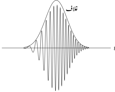
شکل ۱۲.۱۴: چچہاٹ میں گاوسی غلاف کے نیچے بڑھتی تعدد دکھائی گئی ہے۔
