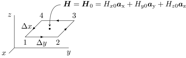
شکل ۱۱.۷: گردش کی تعریف۔
