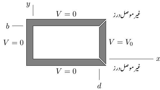
شکل ۶.۳: موصل سطحوں سے گھیرے نطے میں لاپلاس مساوات متعدد اجزاء کے مجموعے سے حاصل ہوتا ہے۔
