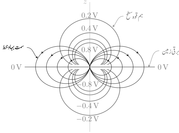
شکل ۴.۱۰: جفت قطب کے ہم قوہ اور سمت بہاؤ خط۔
