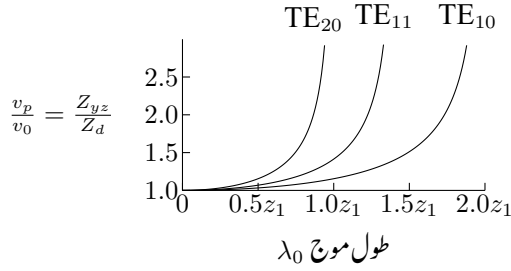
شکل ۱۳.۱۳: مختلف بلند رتبہ امواج کے مستطیلی موج میں دوری رفتار بالمقابل طول موج \lambda_0 ۔
