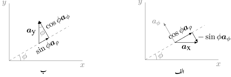
شکل ۱.۲۲: a_x اور a_y کا ٹکلی محدود میں تبادلہ۔
