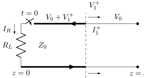
شکل ۱۱.۲۵: ترسیلی تار سے مستطیل پتلا اشارہ حاصل کیا جاسکتا ہے۔
