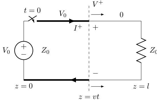
شکل ۱۱.۱: ترسیلی تار میں ابتدائی موج۔
