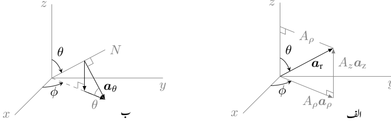
شکل ۱.۳۲: کروی اکائی سمتیات کا کارتیسی نظام میں تبادلہ۔
