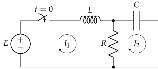
شکل ۴.۲۰: مثال ۹.۷، اور مثال ۸.۰ کا برقی دور۔
