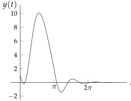
شکل ۶.۲۱: اسپرنگ اور کمیت کا جبری ارتعاش (مثال ۶.۲)۔
