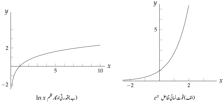
شکل ب. ۱: قوت نمائی تفاعل اور قدرتی لوگار تھم تفاعل
