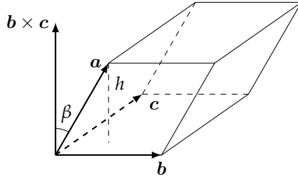
شکل ۷.۲۵: عددیہ سہ ضرب کی جیومیٹریکی معنی۔
