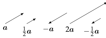
(i) سمتیات کا عددیوں کے ساتھ ضرب۔
