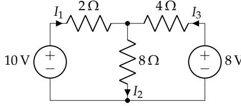
شکل ۸.۳: برقی دور۔ مثال ۸.۳۱
