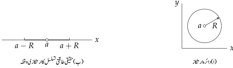
شکل ۱۸.۱: دائرہ اور وقفہ مرکز اور وقفہ مرکز
