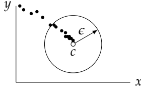
شکل ۱۷.۱: مرکوز مخلوط ترتیب
