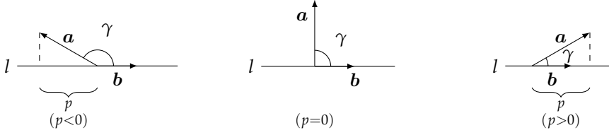
شکل ۷.۱۳: b کی سمت میں a کا جزو۔
