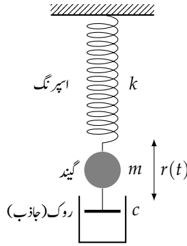
شکل ۲.۲۱: اسپرنگ اور گیت کے نظام کی جبری ارتعاش۔
