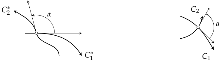
شکل ۱۵.۱۰: منحنیات C_1 اور C_2 کا محافظ زاویہ نقش کشی میں عکس بالترتیب C_1^* اور C_2^* ہے۔
