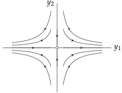
(ا) نظام ۴.۵۱ کے خط حرکت۔ (نقطہ زین)
