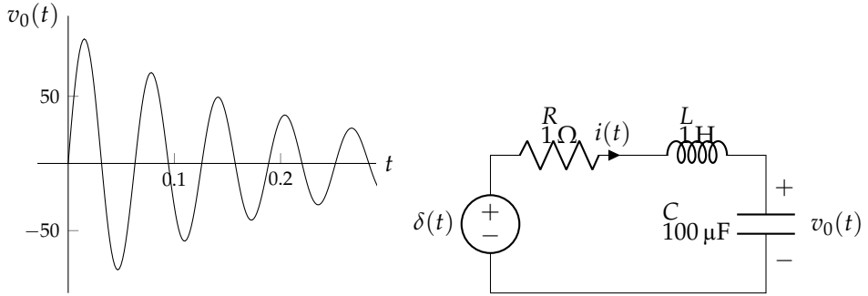
شکل ۶.۲۰: سلسلہ واردور (مثال ۶.۲۳)۔
