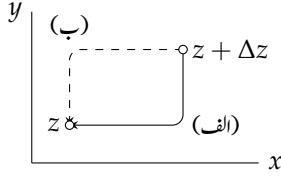
شکل ۱۰.۱۴: راہ (مساوات ۱۴.۴۱)
