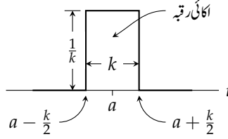
شکل ۶.۱: ڈیلٹائی فنکشن۔
