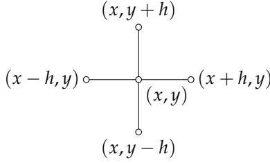
شکل ۳.۴: (۲۳.۲۸ مساوات اور ۲۳.۲۹ مساوات میں مستعمل نقطے
