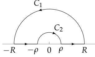
شکل ۱۹.۱۱: شکل ۱۹.۱۱ کے برائے مثال ۱۹.۱۱
