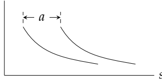
شکل ۶.۴: منتقلی کا پہلا مسئلہ، s محور پر منتقلی
