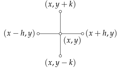
شکل ۳.۳: (۲۳.۲۶ مساوات اور ۲۳.۲۷ مساوات میں مستعمل نقطے
