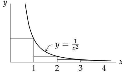
شکل ۱۷.۹: تسلسل ۱، ۲، ۳، ۴ کا ریکٹانگل
