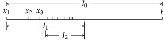
شکل ۱۷.۴: شکل برائے ثبوت مسئلہ ۱۷.۱۰
