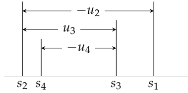
شکل ۱۷.۸: ثبوت مسئلہ ۱۷.۱۱ (لیبنٹز پرکھ)
