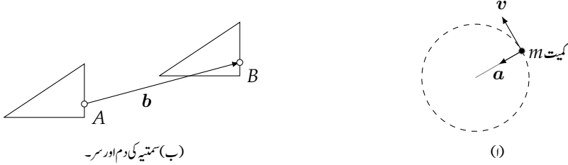
شکل ۱۔ سمتیہ کی تفصیل۔
