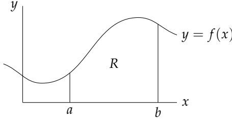
شکل ۲۱.۷: قطعی تکمیل کی جیومیٹریکی معنی
