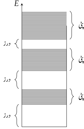
شکل ۵.۵: دوری محفہ کی اجازتی توانائیاں بنیادی طور پر استمراری پٹیاں پیدا کرتی ہیں۔
