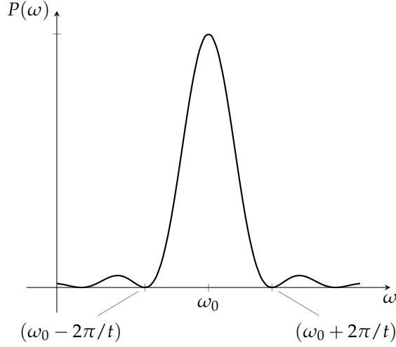
شکل ۹.۲: تویلی احتمال بالمقابل متحرک تعدد (مساوات ۹.۲۸)۔
