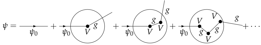
شکل ۱۱.۱۳: بارن تسلسل (مساوات ۱۱.۱۰۱) کی نظری مفہوم۔
