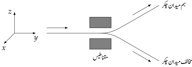
شکل ۴.۱۱: شرن و گرلاخ آلہ۔
