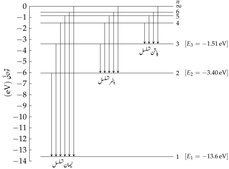
شکل ۷.۴: ہائیڈروجن طیف میں سطحوں توانائی اور تحویلات۔
