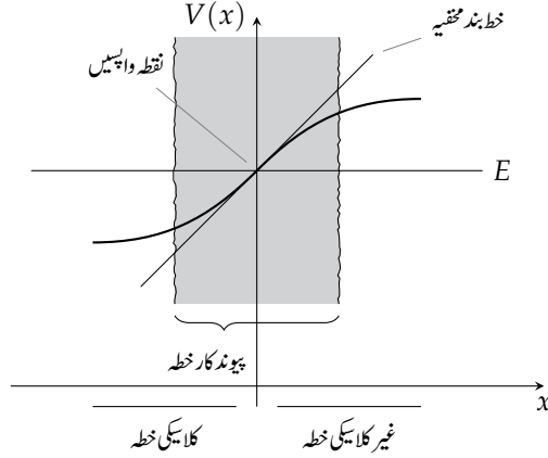
شکل ۸.۴: دائیں ہاتھ نقطہ واپسیں کو وضاحت سے دکھایا گیا ہے۔
