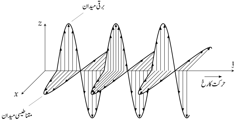
شکل ۹.۳: برقی طبعی موج۔
