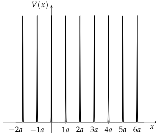
شکل ۵.۵: ڈیراک کنگھی (مساوات ۵.۵)۔
