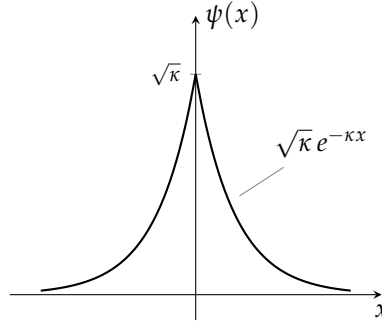
شکل ۲.۱۴: ڈیلٹا تفاعل محفئہ (مساوات ۲.۱۲۲) کے لئے مقید حال تفاعل موج۔
