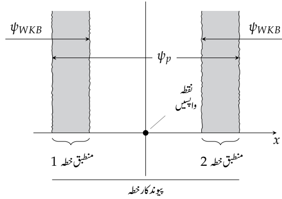
شکل ۸.۹: پیوندی خطہ اور دو منطقہ خطہ۔
