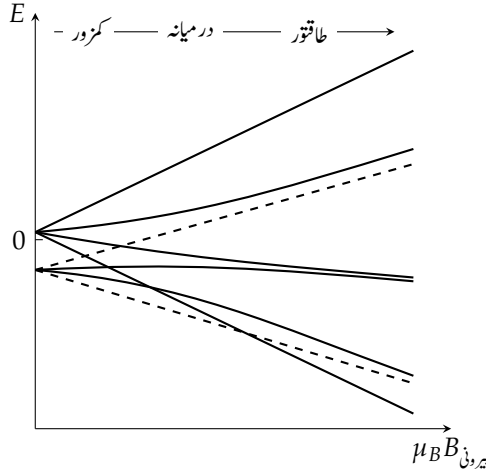
شکل ۶.۱۲: کمزور، درمیانہ اور طاقتور میدان میں ہائیڈروجن کے n = 2 حال کا زیمان بنواری۔
