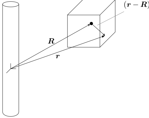
شکل ۱۰.۱۲: مختلف V(r - R) ایک ذرے کو ڈبے میں مقید کیے ہوئے ہے۔
