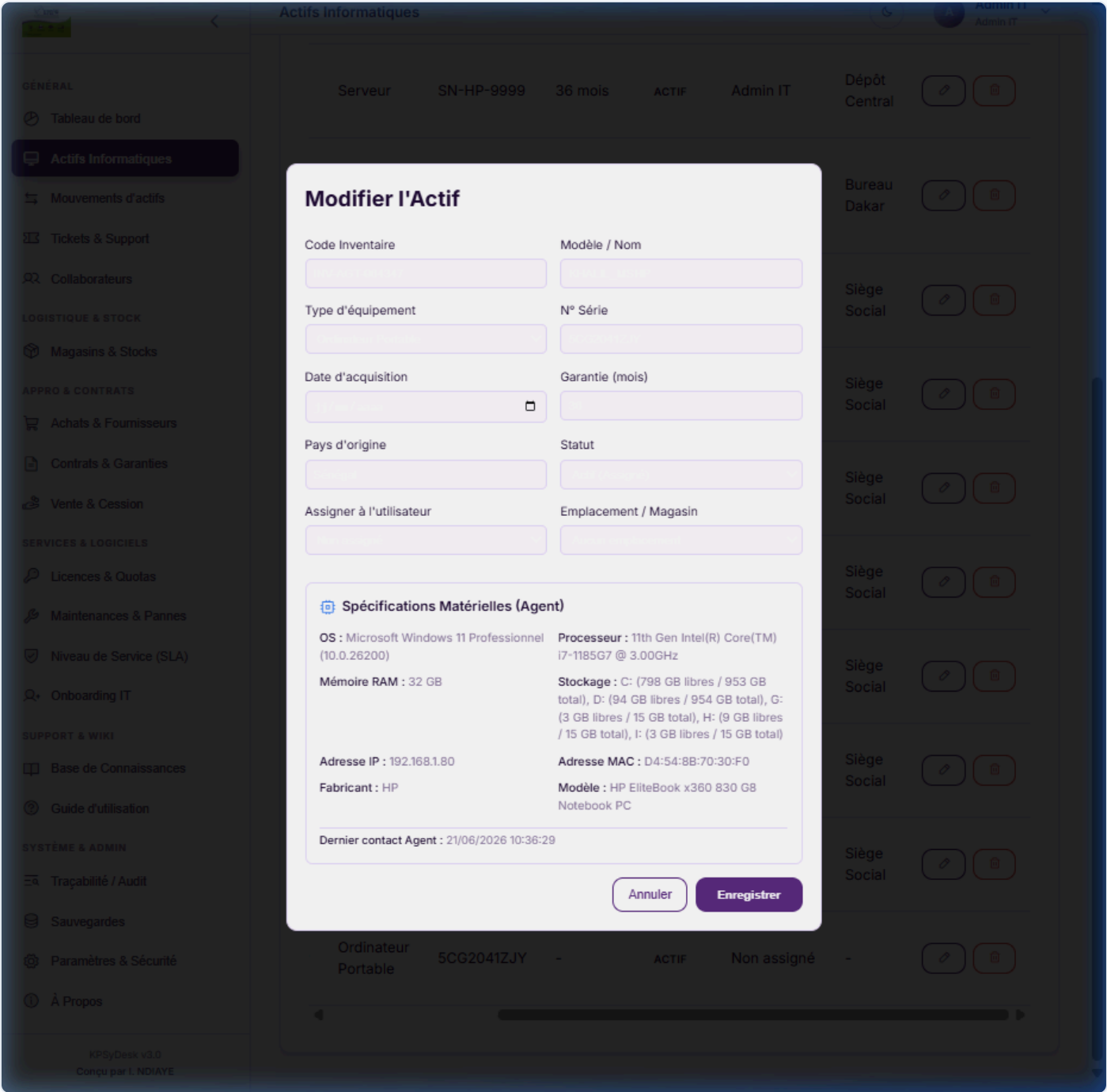
Figure 6 : Encart "Spécifications Matérielles (Agent)" apparaissant au bas d'un équipement après enrôlement automatique.
