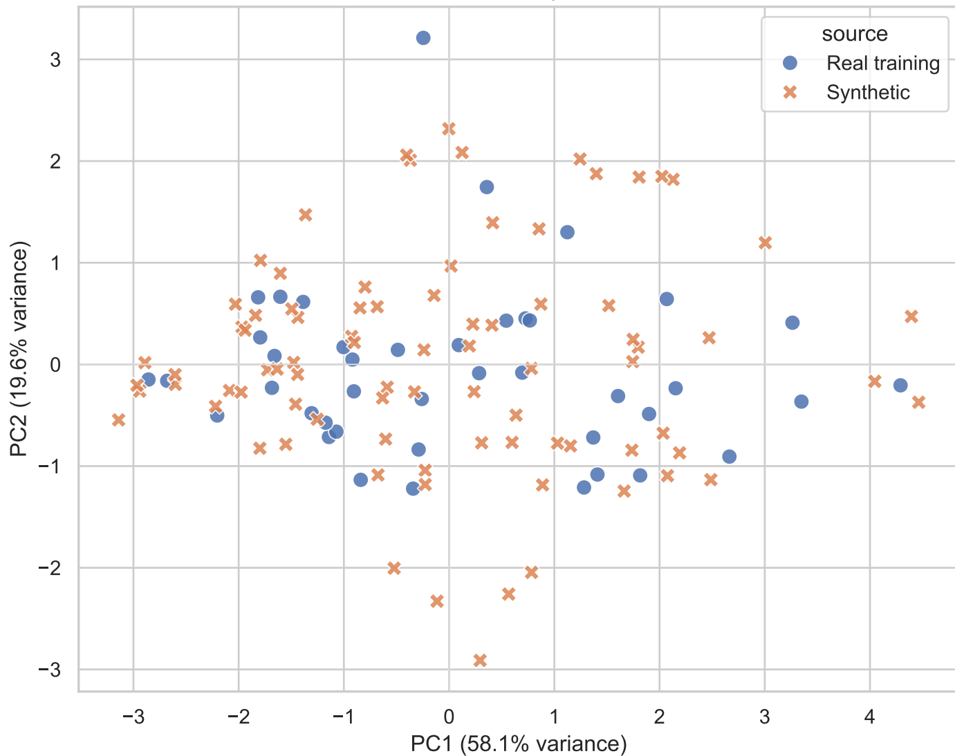
Clearance real-vs-synthetic PCA
