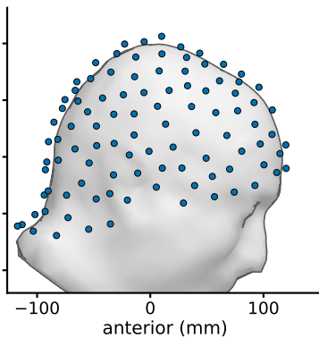
C Dense OPM array
