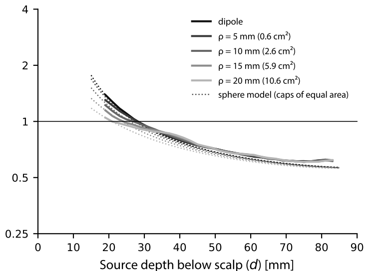
A Median \text{SNR}_{\text{OPM}} / \text{SNR}_{\text{SQUID}}
