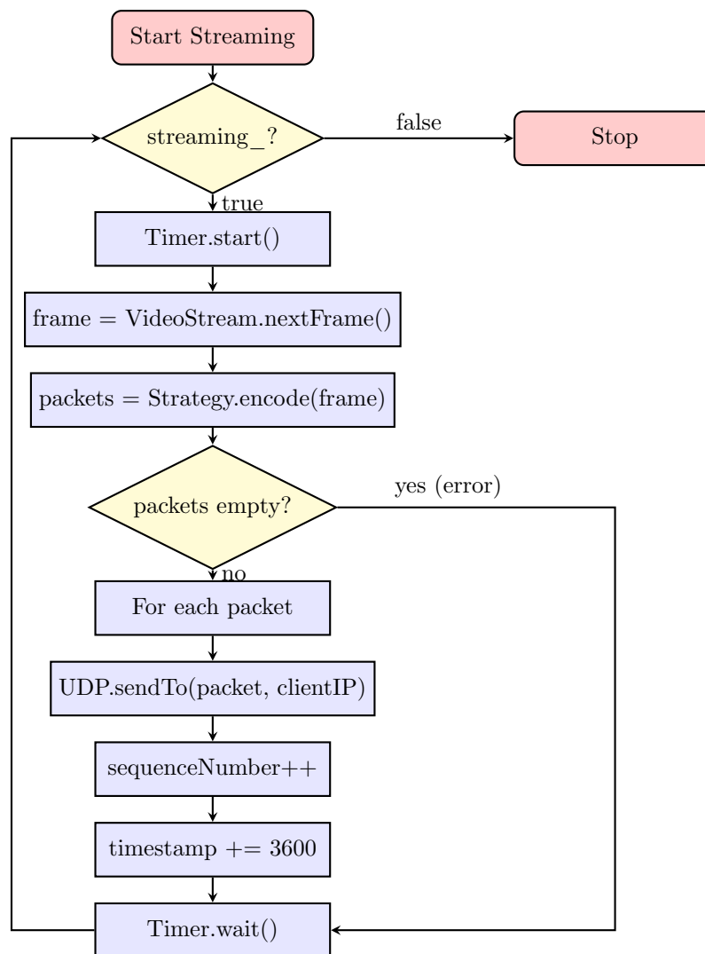
Figure 7: Flowchart thuật toán Server Streaming Loop
