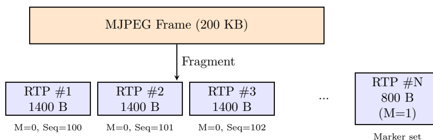
Figure 8: Fragmentation một frame MJPEG thành nhiều RTP packets
