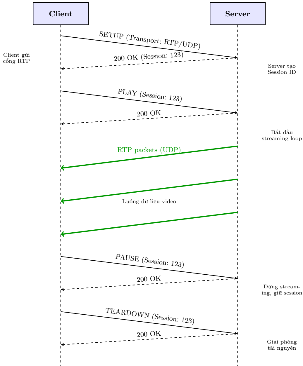
Figure 6: Sequence diagram của một phiên RTSP/RTP hoàn chỉnh
