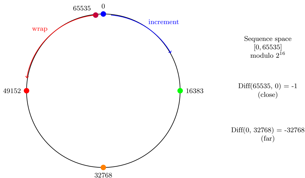
Figure 10: Không gian sequence number 16-bit và wrap-around
