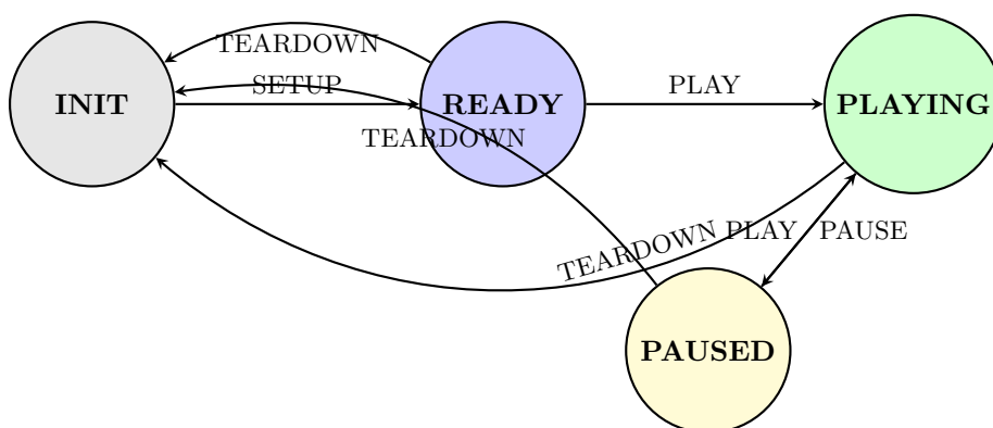
Figure 5: Máy trạng thái RTSP với các chuyển đổi hợp lệ
