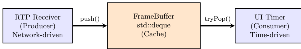
Figure 12: Mô hình Producer-Consumer của FrameBuffer
