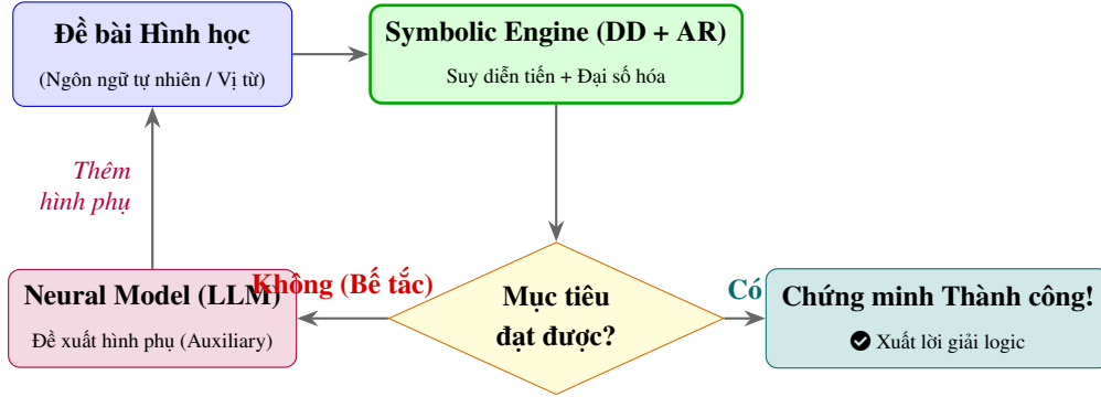
Hình 1.1: Sơ đồ vòng lặp cộng sinh Neuro-Symbolic của AlphaGeometry (Google DeepMind).
