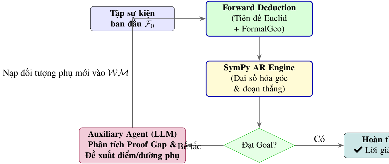
Hình 3.1: Quy trình phối hợp toàn diện giữa Suy diễn tiến, SymPy AR và Tác tử Sinh hình phụ.
