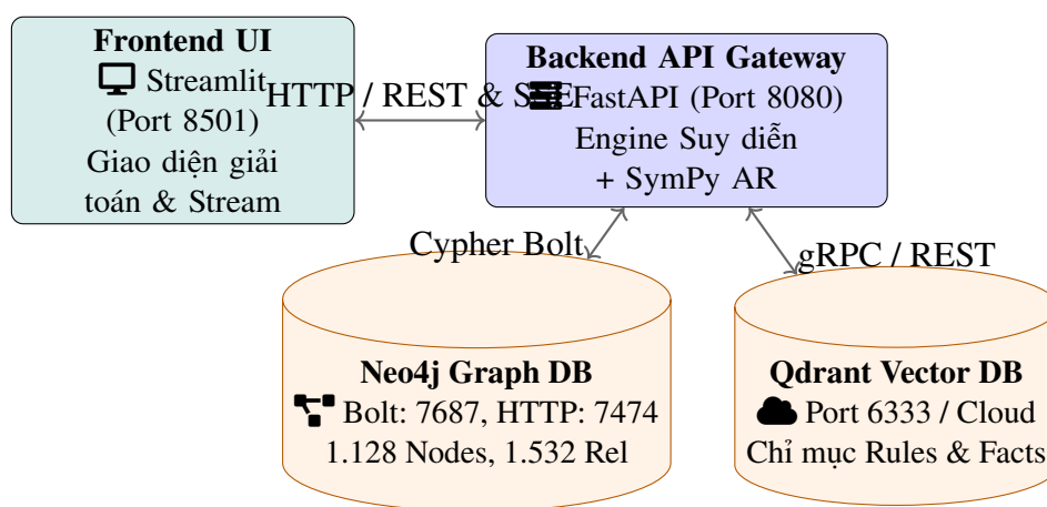
Hình 4.1: Sơ đồ kiến trúc Microservices Docker của hệ thống AlphaGeometry-IMO.
